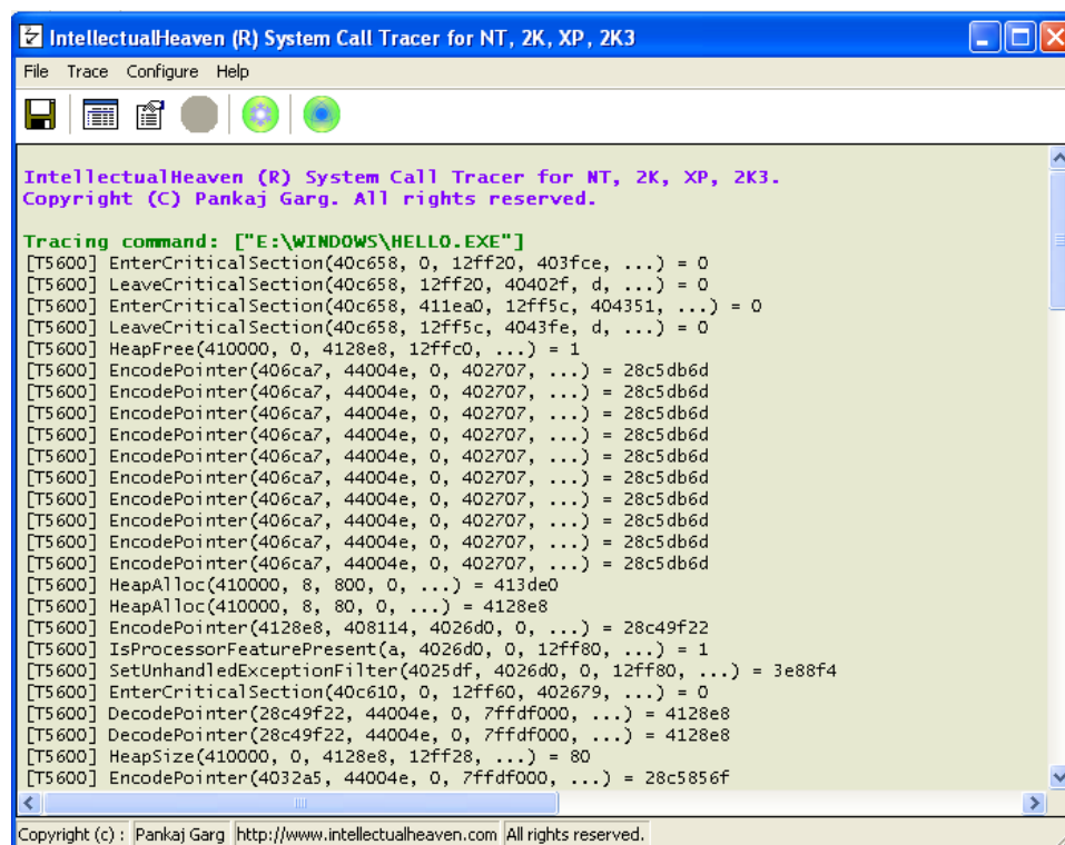
Figura 22.- Visualización del programa StraceNT
