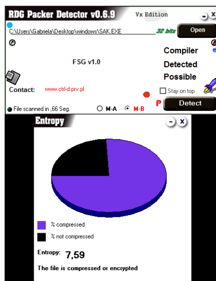
Figura 32.- Análisis con RDG Packer Detector
