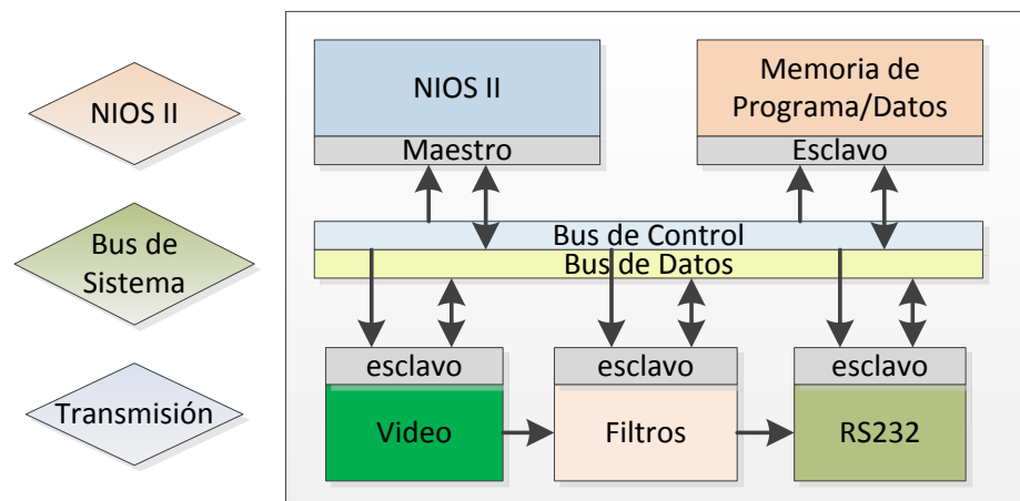
Figura 2.12 - INTERCONEXIÓN DE PERIFÉRICOS CON LA RED AVALON [11]
