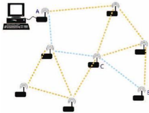
Figura 2.23 - RED MESH IMPLEMENTADA CON MÓDULOS XBEE CARACTERÍSTICAS [22]
