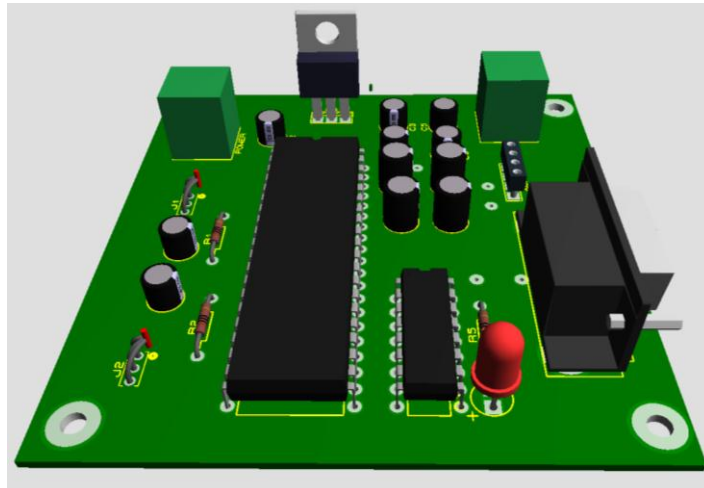
VISTA EN 3D DEL MODULO TRANSMISOR
