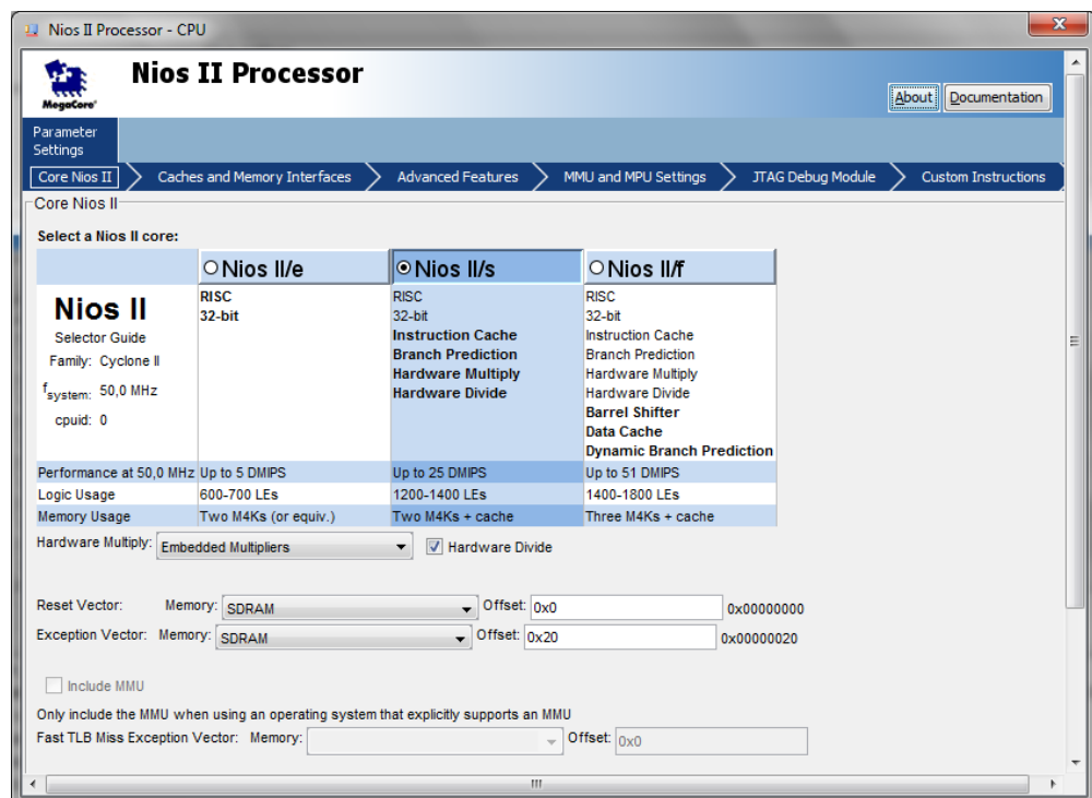
Figura 3.9 - CONFIGURACIÓN DEL MICROPROCESADOR NIOS II
