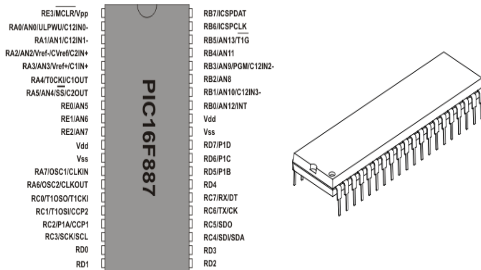
Figura 2.15 - EMPAQUETADO TIPO DIP PIC 16F887 [14]
