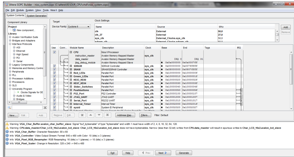
Figura 3.8 - DISEÑO DEL MÓDULO RECEPTOR EN SOPC BUILDER
