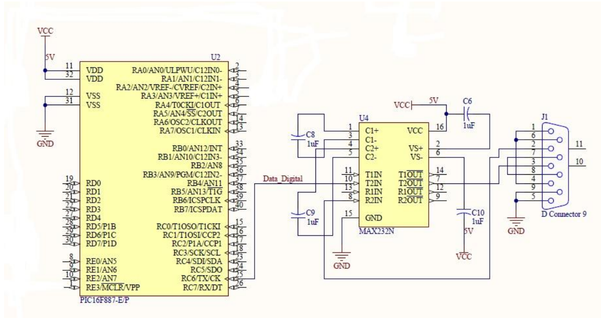
Figura 3.7 - ETAPA DE TRANSMISIÓN
