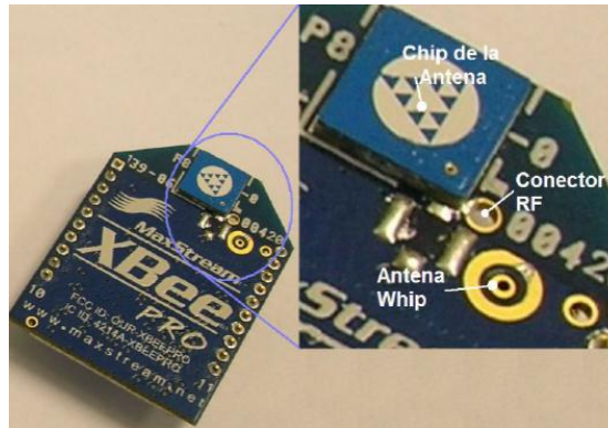
Figura 2.22 - ELEMENTOS DEL XBEE [21]
