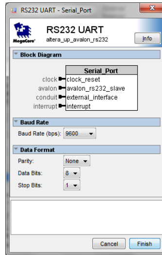
Figura 3.12 - CONFIGURACIÓN DEL MÓDULO UART
