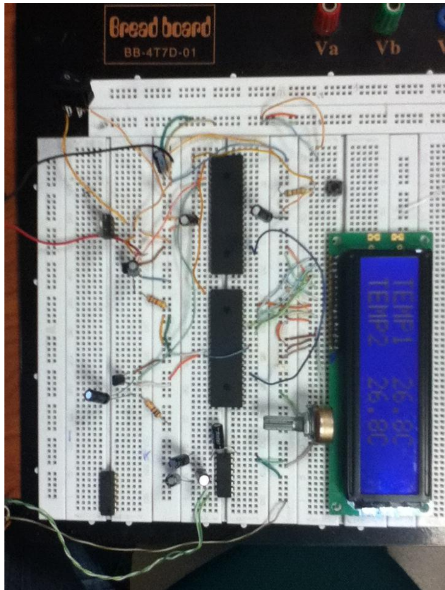
Figura 3.17 - TRANSMISIÓN DE SEÑAL
