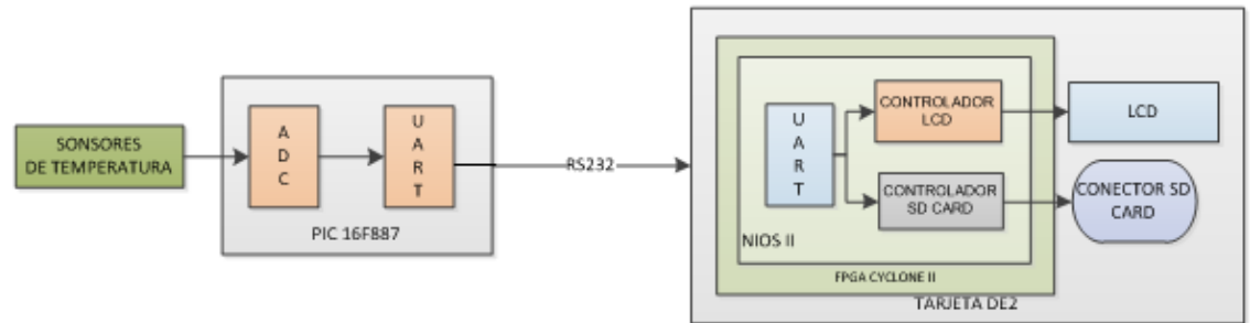
Figura 3.2 - DIAGRAMA DE BLOQUES DEL DATALOGGER
