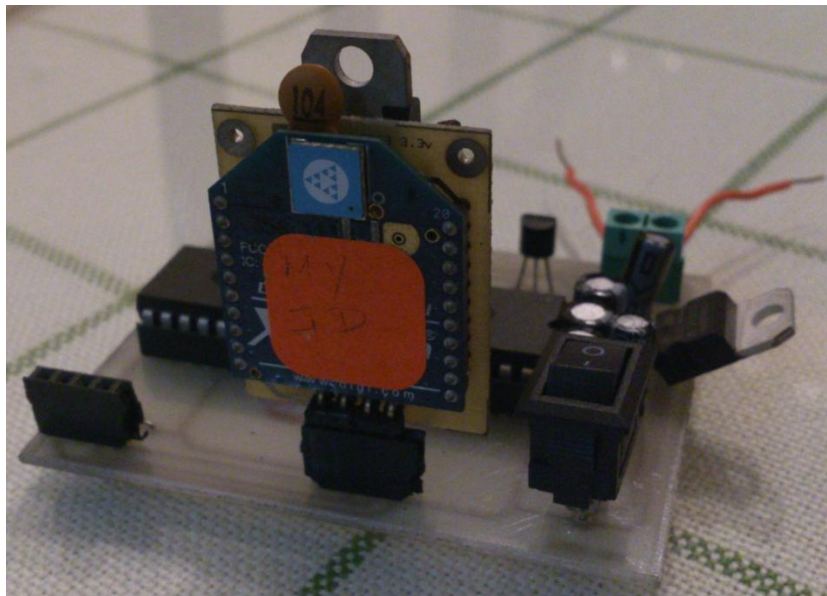
Figura 3.20 - MÓDULO DE COMUNICACIÓN INALÁMBRICA
