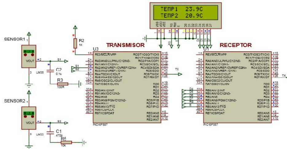
Figura 3.16 -CIRCUITO SIMULADO EN PROTEUS
