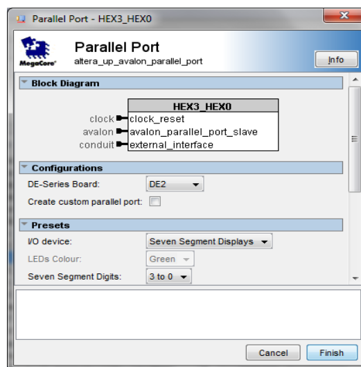
Figura 3.10 - DISPLAYS DE 7 SEGMENTOS
