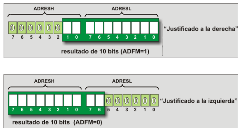
Figura 2.17 - REGISTROS DE ALMACENAMIENTO DE LOS DATOS CONVERTIDOS [16]
