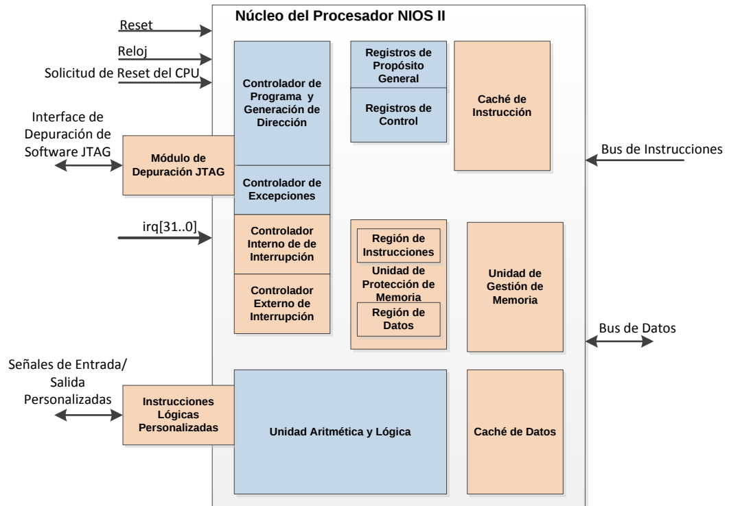
Figura 2.10 - ESTRUCTURA DEL MICROPROCESADOR NIOS II [9]
