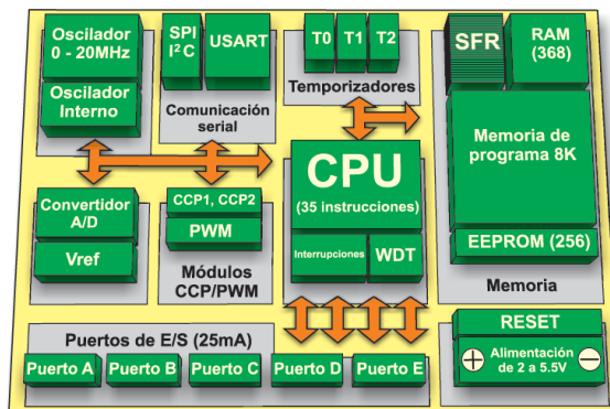
Figura 2.13 - DIAGRAMA DE BLOQUES PIC 16F887 [12]
