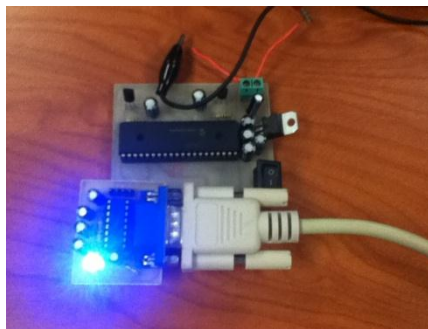
Figura 4.4 - MÓDULO TRANSMISOR
