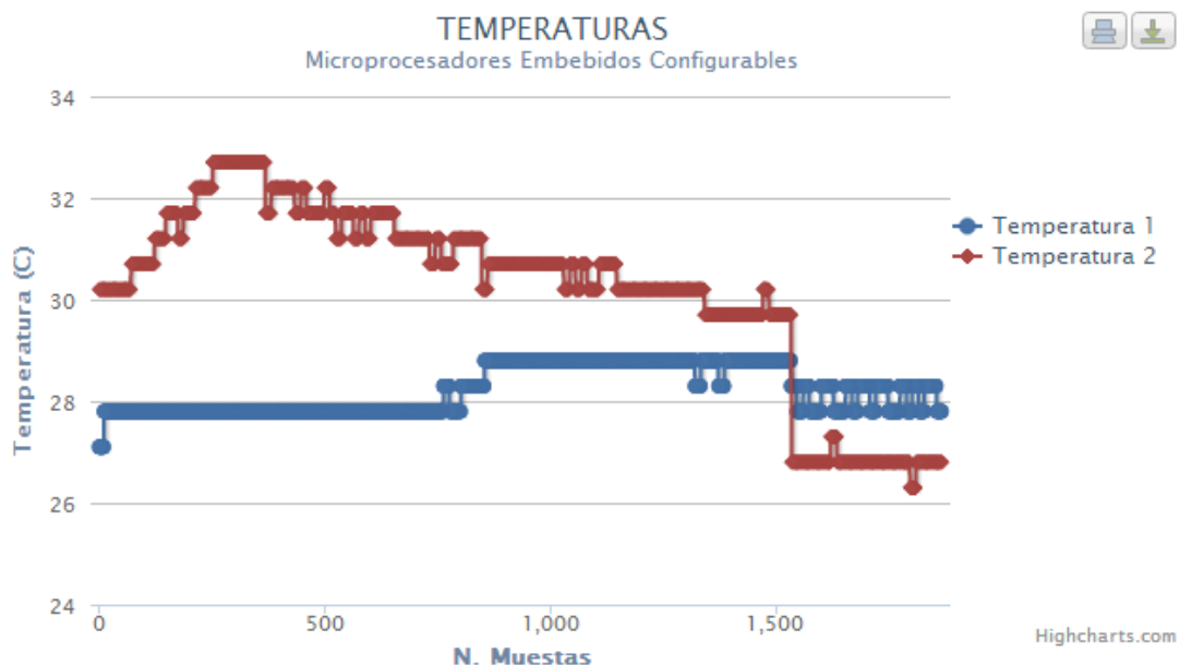
Figura 4.6 - GRAFICA TEMPERATURA VS NÚMERO DE MUESTRAS
