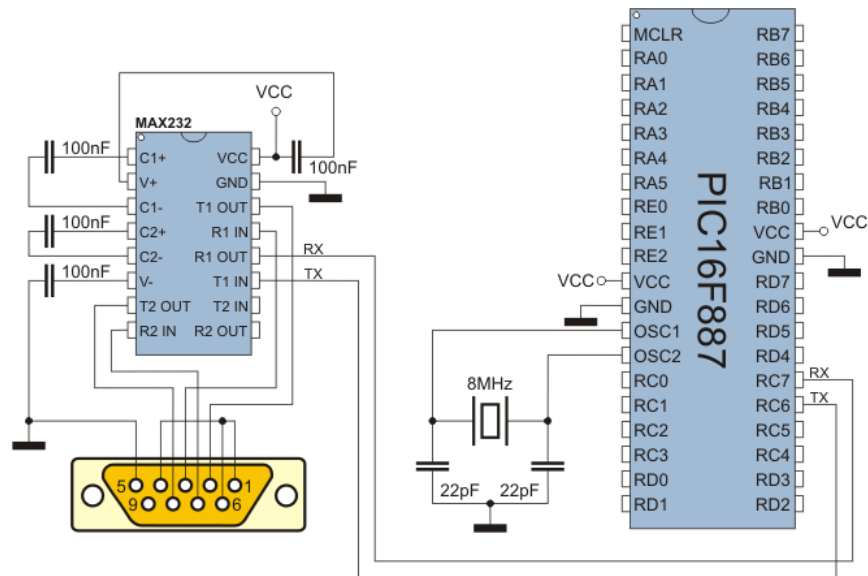
Figura 2.20 - ESQUEMÁTICO DE CONEXIÓN RS232 [19]
