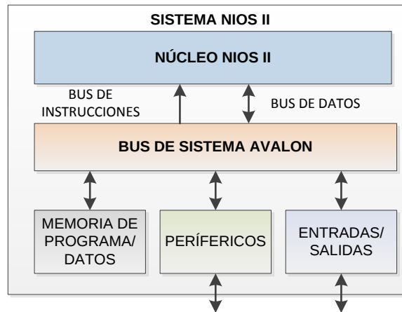
Figura 2.9 - SISTEMA BASADO EN EL MICROPROCESADOR NIOS II [8]
