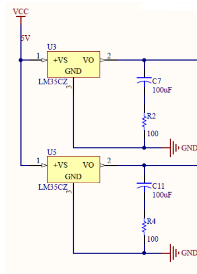
Figura 3.5 - SENSORES DE TEMPERATURA LM35
