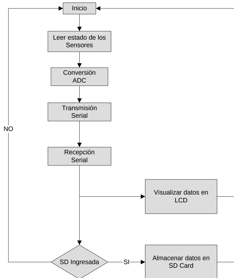
Figura 3.1 - DIAGRAMA FUNCIONAL DE LA SOLUCIÓN IMPLEMENTADA
