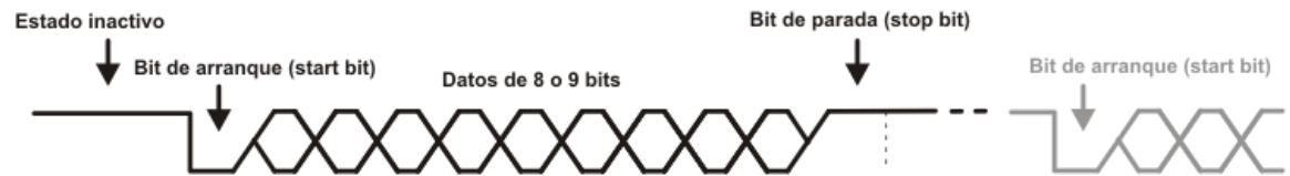
Figura 2.19 - MÉTODO DE TRANSMISIÓN SERIAL [18]
