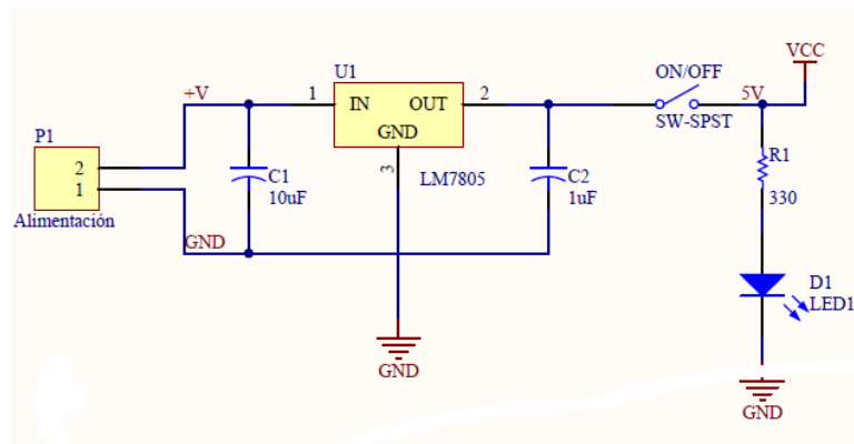
Figura 3.4 - ETAPA DE ALIMENTACIÓN
