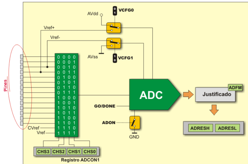
Figura 2.16 - MÓDULO ADC PIC 16F887 [15]
