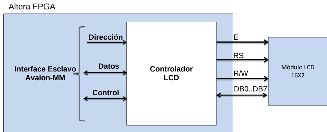
Figura 2.3 - DIAGRAMA DE CONEXIÓN DEL MÓDULO LCD16X2 [3]
