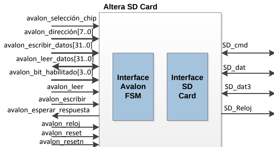
Figura 2.6 - MÓDULO SDCARD [5]
