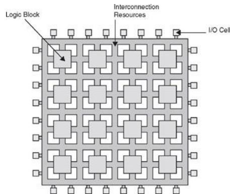
Figura 2.7 - ESTRUCTURA DE UNA FPGA [6]
