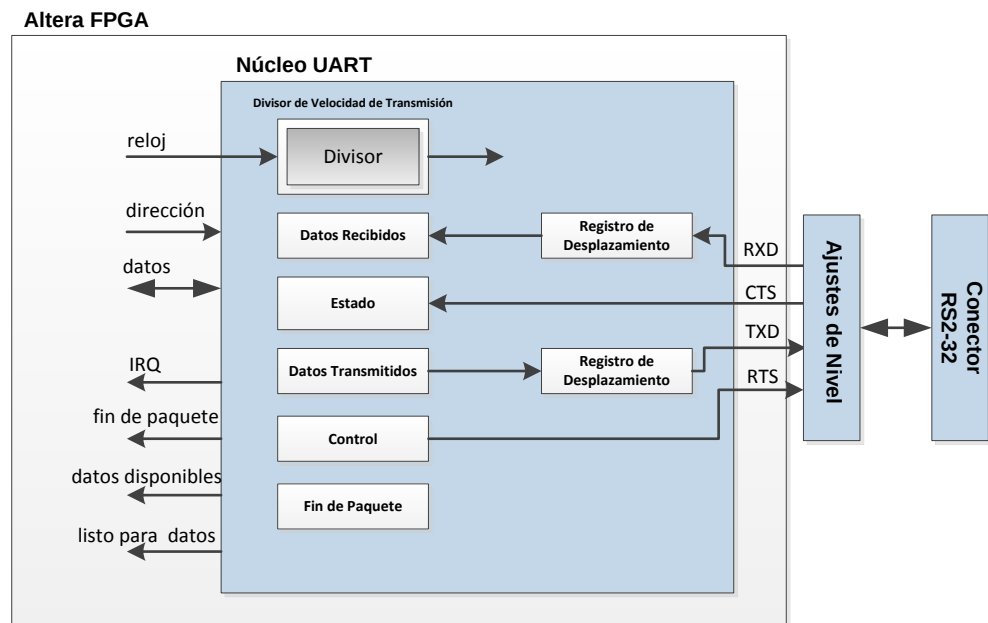
Figura 2.4 - MÓDULO UART [4]
