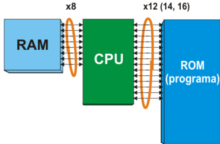
Figura 2.14 - ARQUITECTURA PIC 16F887 [13]
