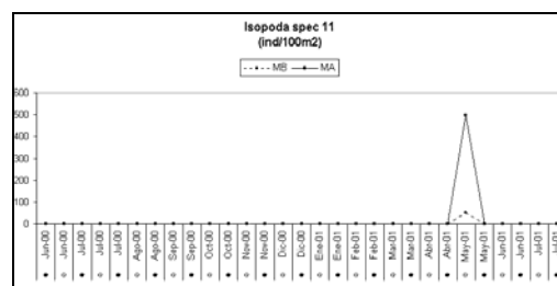
Figura 48: Isopoda spec 11
