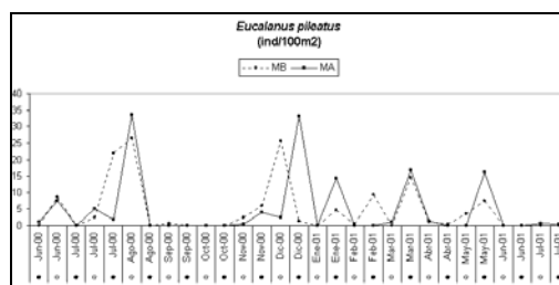
Figura 44: Eucalanus pileatus
