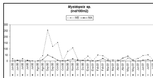
Figura 54: Mysidopsis spec 1 .
