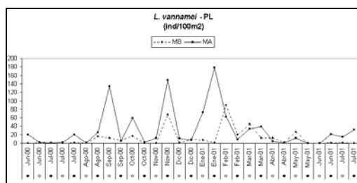
Figura 55: L. vannamei
