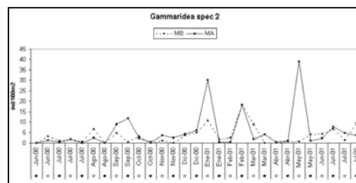
Figura 46: Gammaridea spec 2
