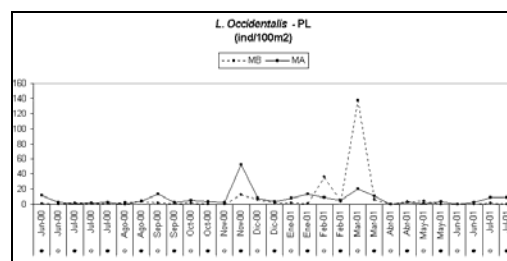
Figura 56: L. occidentalis
