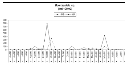
Figura 52: Bomwmaniela spec 1.
