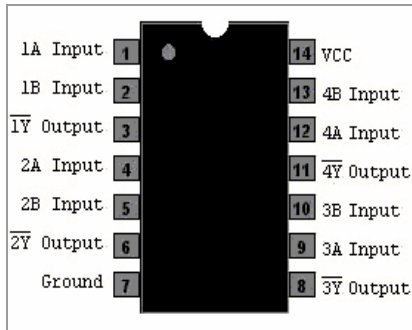
Figura 1. Integrado 7400
