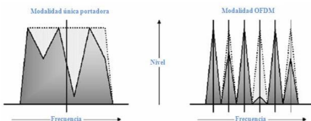
Figura1.12.- Modalidad única portadora y Modalidad OFDM.
