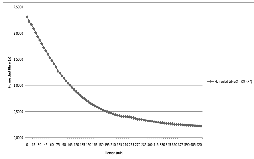
Figura 2.4 HUMEDAD LIBRE VS TIEMPO
