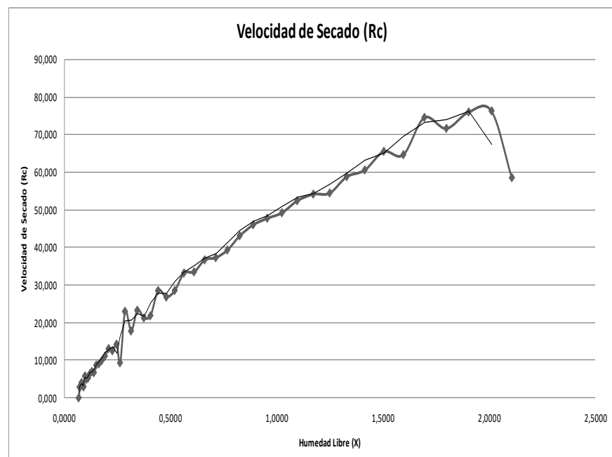
Figura 2.5 VELOCIDAD DE SECADO VS HUMEDAD LIBRE
