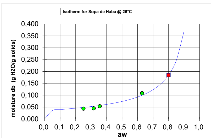
FIGURA 3.1 ISOTERMA DE ADSORCIÓN DE LA SOPA
