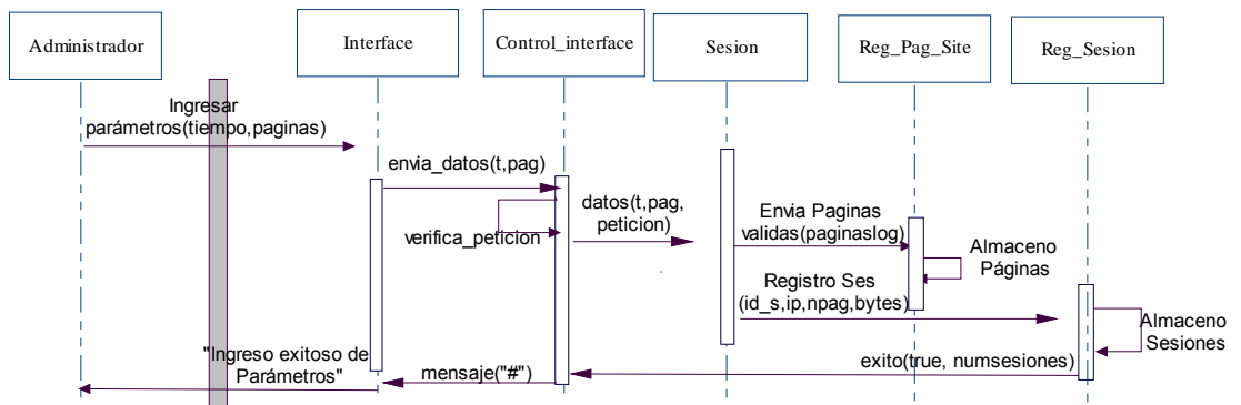
Figura C.8 Escenario 2.4: Ingreso exitoso de parámetros para procesamiento
