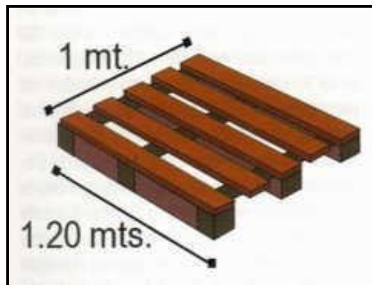
FIGURA 4.2. PALLETS INTERCAMBIABLES DE MADERA
