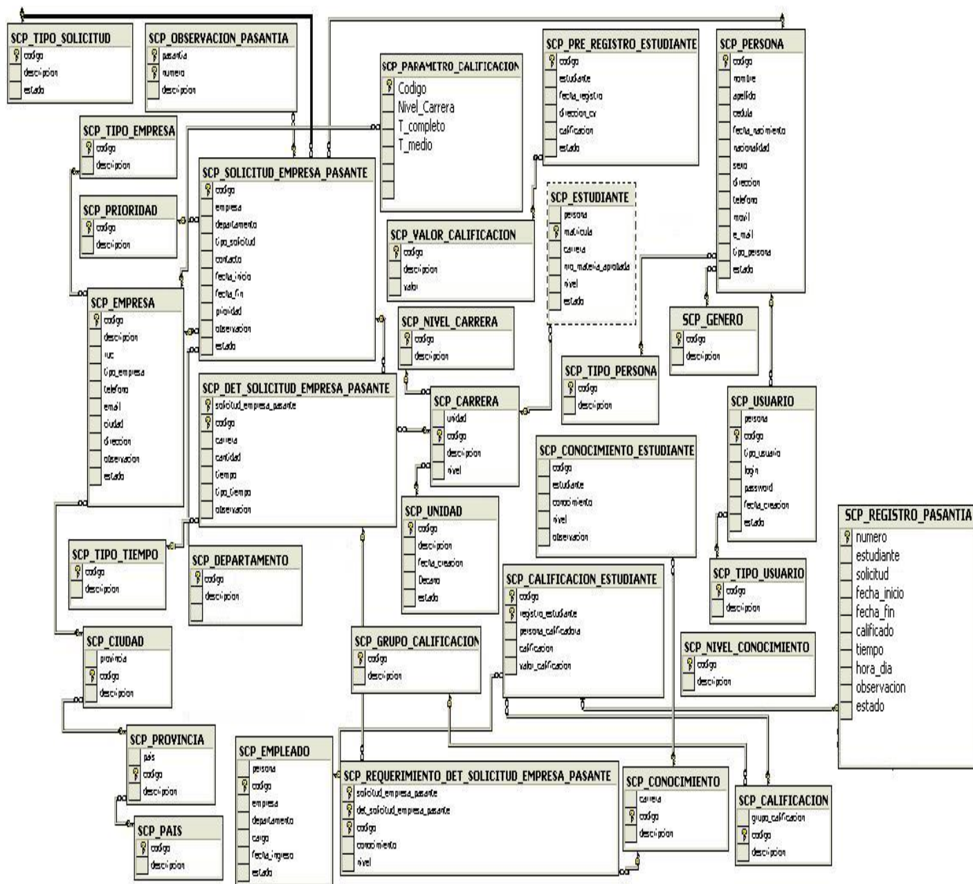
Ilustración 5-1 MODELO ENTIDAD RELACIÓN
