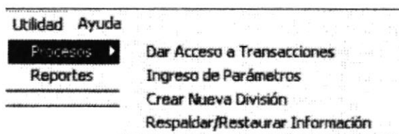
Fig. 1 Menú Utilidad
