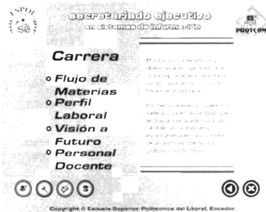
Imagen 4.23. Página Carrera.
