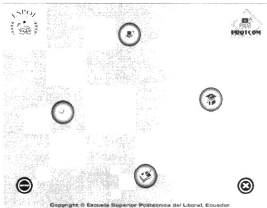
Imagen 3.14. Animación 1
