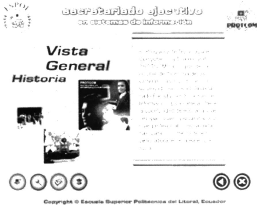
Imagen 4.11. Página Historia.
