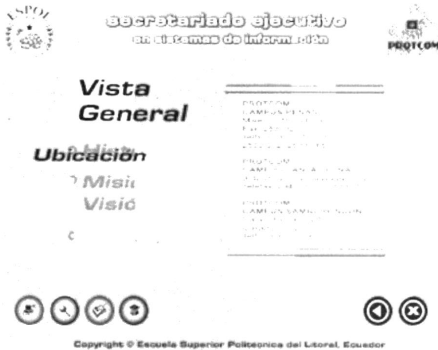
Imagen 3.16. Animación 3
