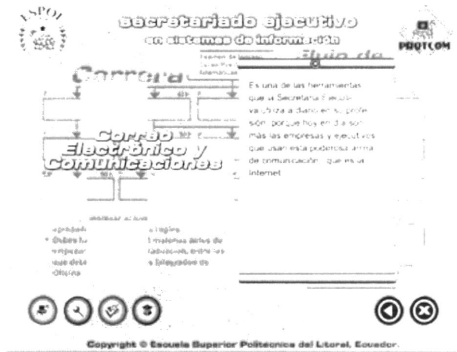
Imagen 4.33. Correo Electrónico.
