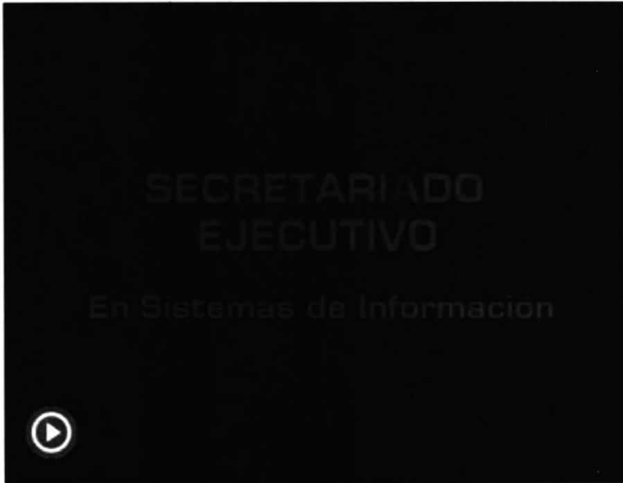
Imagen 4.4 Secuencia 4
