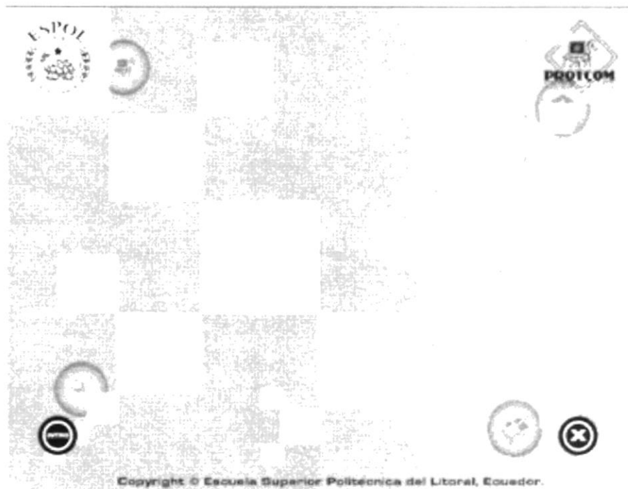
Imagen 3.15. Animación 2
