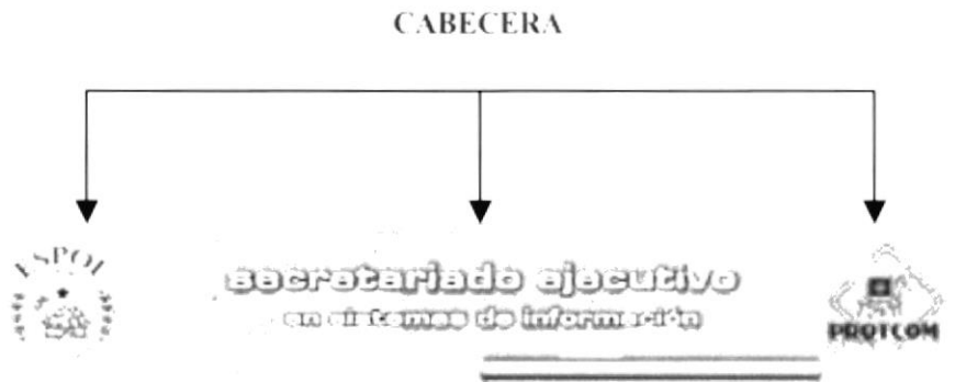
Imagen 3.2. Cabecera.
