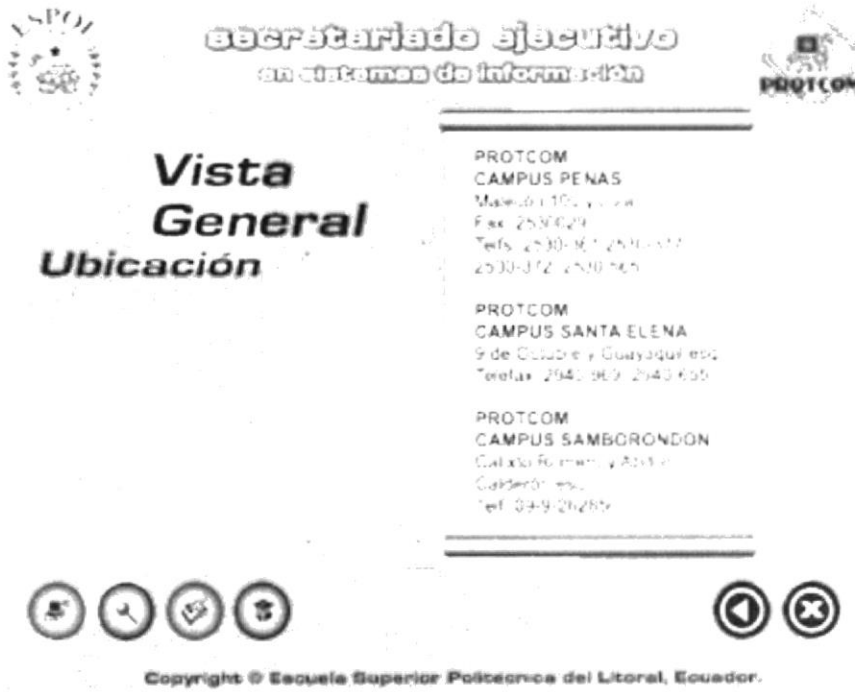
Imagen 4.14. Página Ubicación
