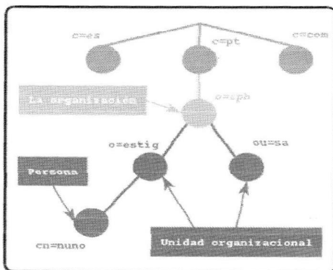
Figura 2. Árbol del directorio LDAP (nombramiento de Internet)
