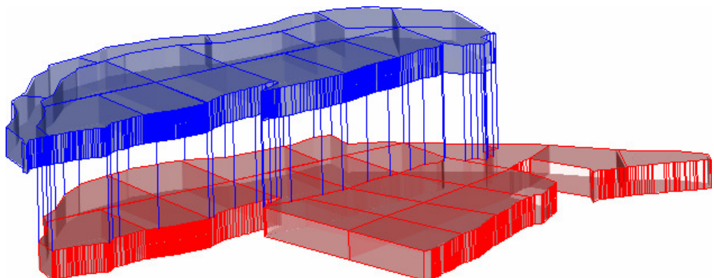
Fig. 5.18. Vista en perspectiva 3-D del nivel 1 y 2
