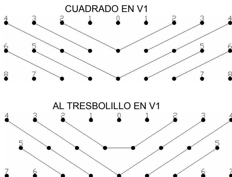
Fig. 4.13. Secuencias de encendido (Hagan, 1975)
