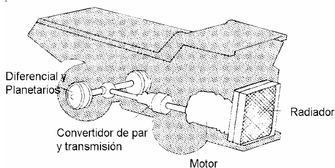
TREN DE TRANSMISION MECANICA
