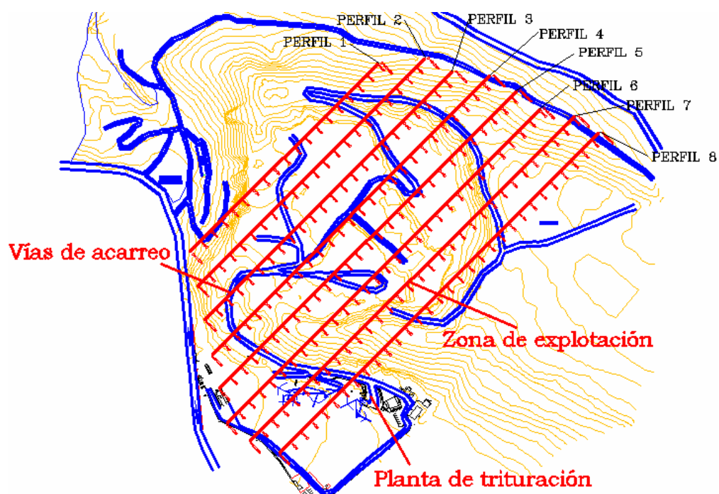
Fig. 5.3. Ubicación en planta de los perfiles topográficos
