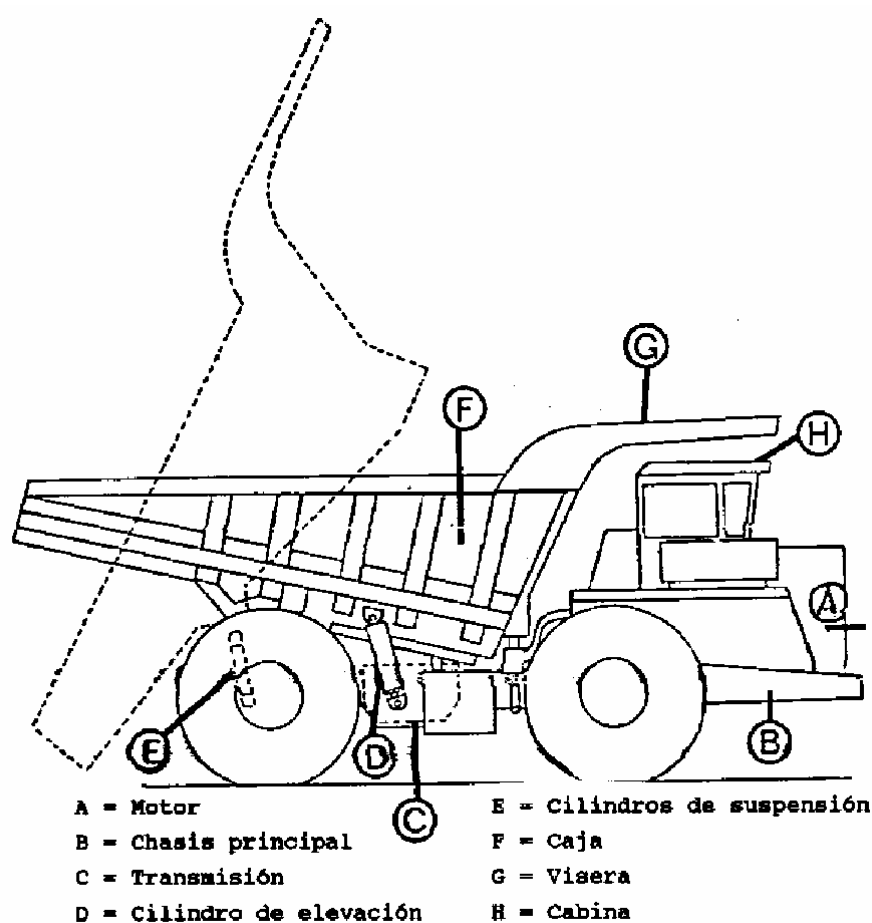
Fig. 4.18. Volquete
