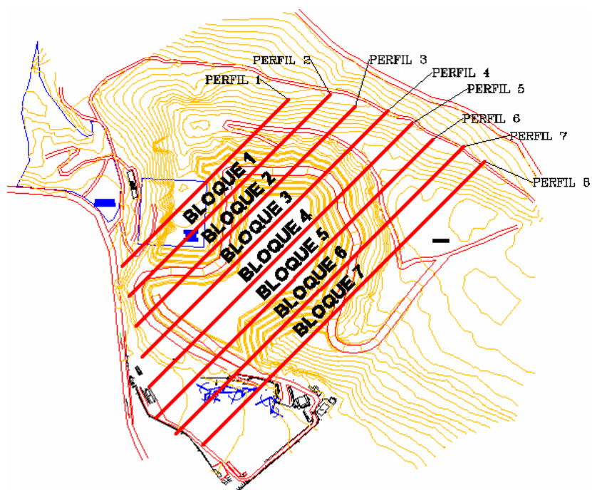
Fig. 5.2. Perfiles topográficos
