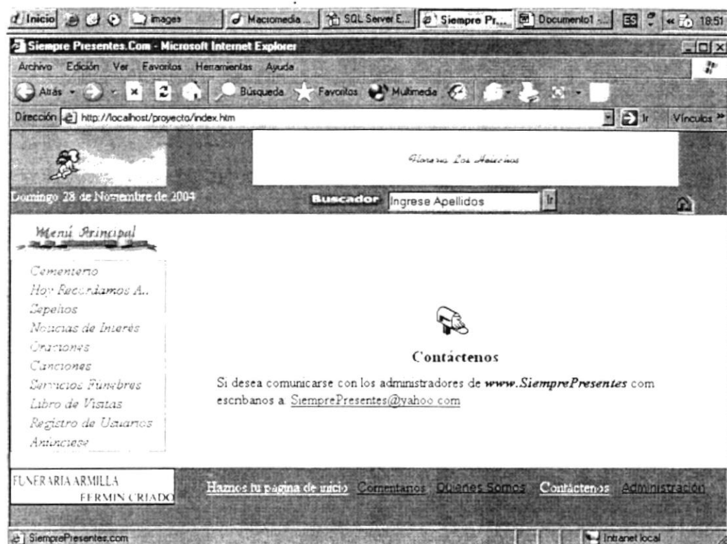
Figura 4.18 Pantalla contáctenos
