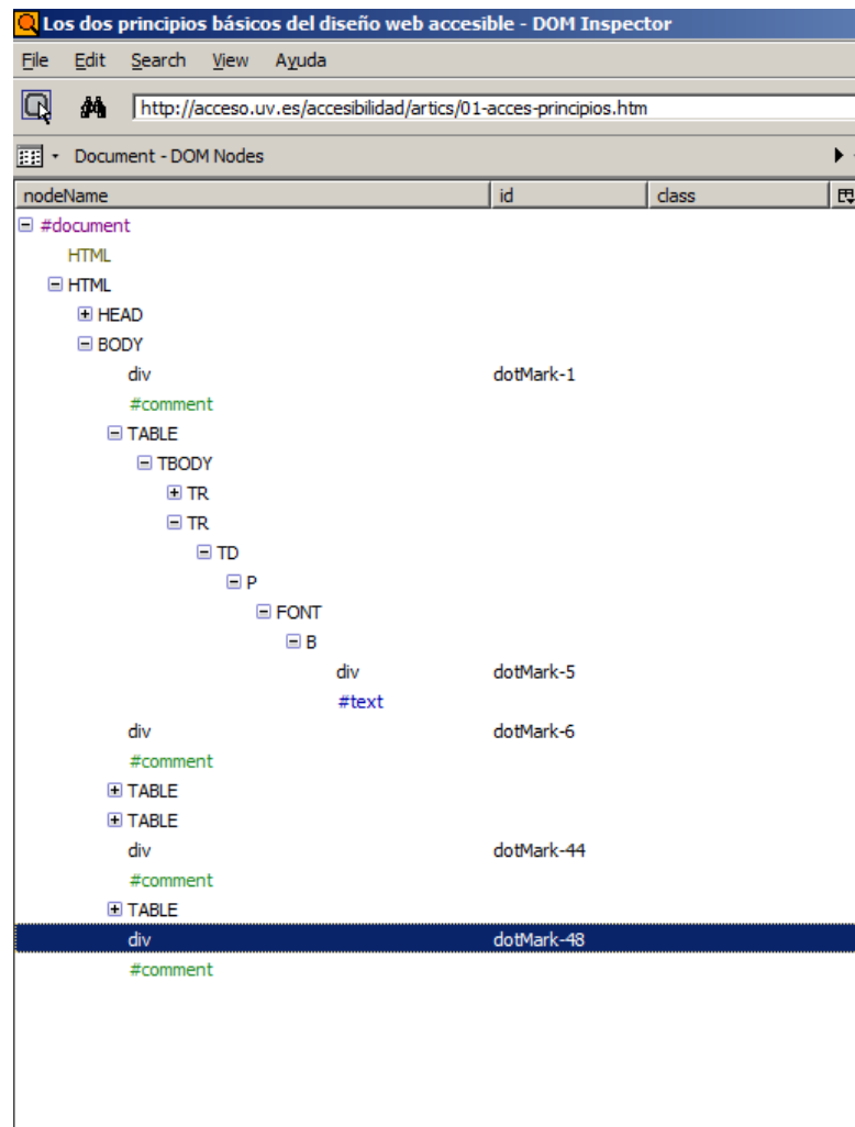
Figura 4.2: Estructura DOM de página con elementos dotMark-##
