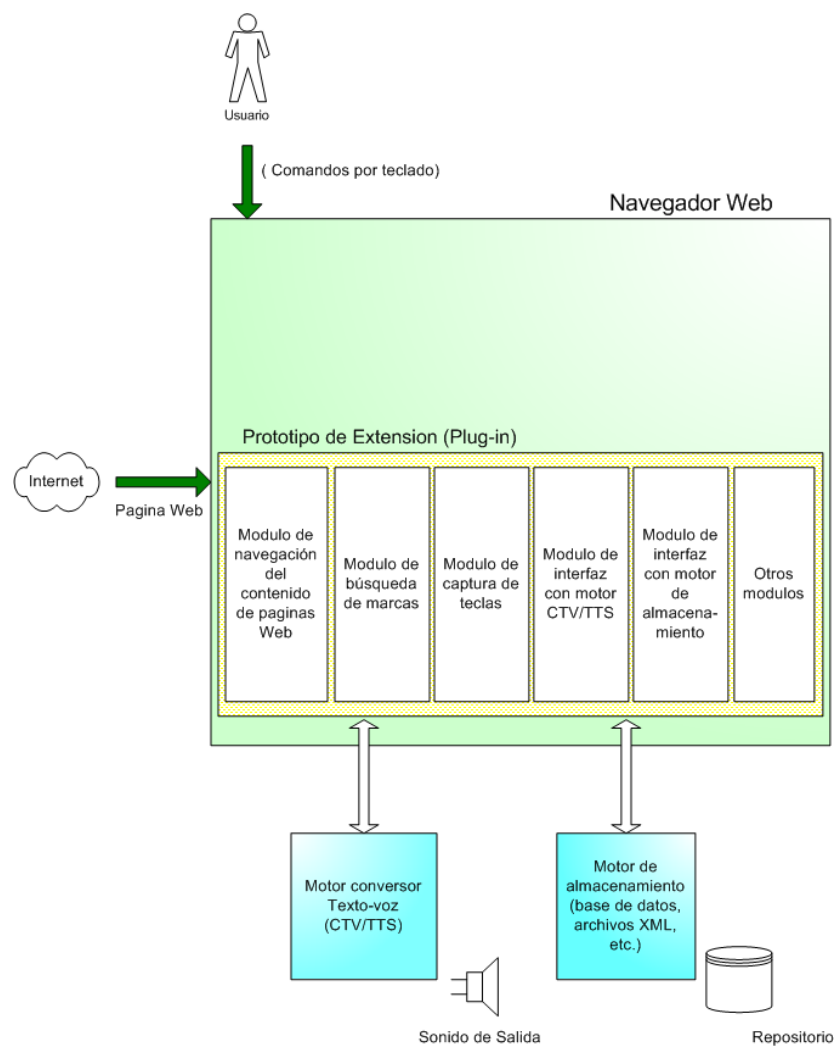
Figura 3.1: Módulos que conforman el prototipo y su interacción
