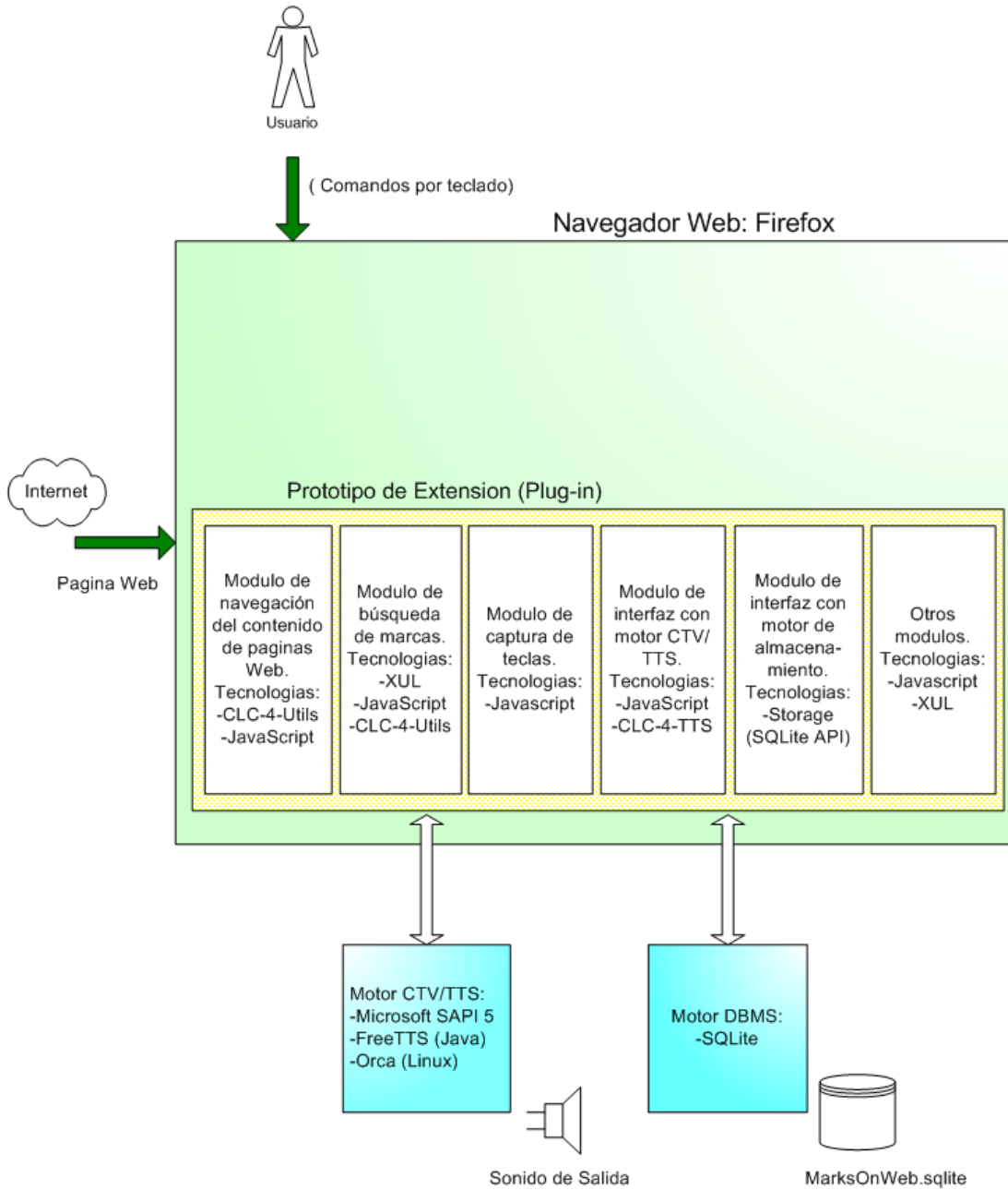
Figura 4.1: Tecnologías utilizadas en sistema de marcas
