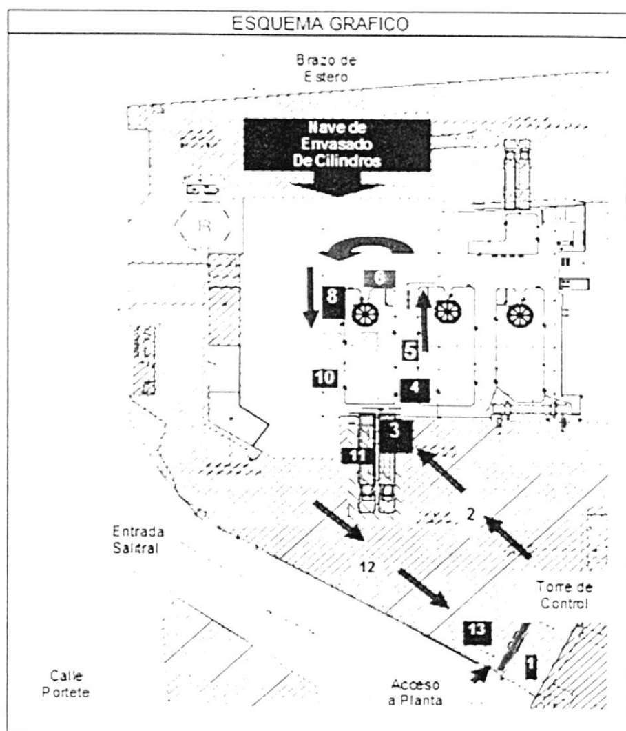
FIGURA 3.3. DIAGRAMA DE RECORRIDO
