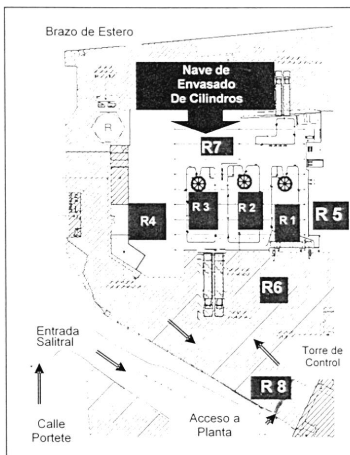
FIGURA 4.27. PUNTOS DE MEDICIÓN DE NIVELES DE RUIDO
