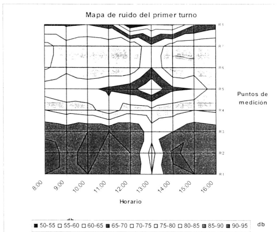
FIGURA 4.28. MAPA DE RUIDO DEL PRIMER TURNO
