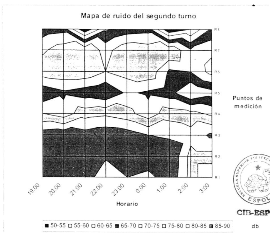
FIGURA 4.29. MAPA DE RUIDO DEL SEGUNDO TURNO
