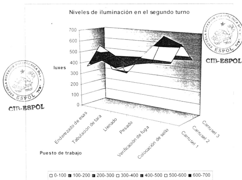
FIGURA 4.31. GRÁFICO DE SUPERFICIE SEGUNDO TURNO
