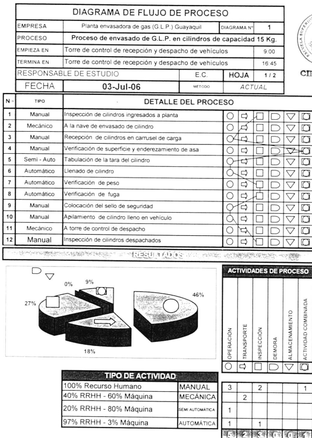
FIGURA 3.2. DIAGRAMA DE PROCESO
