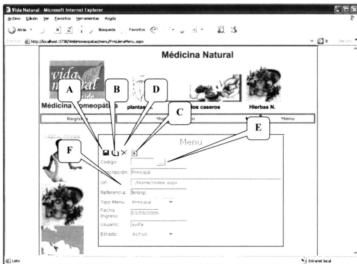
Figura 37. Página Menú
