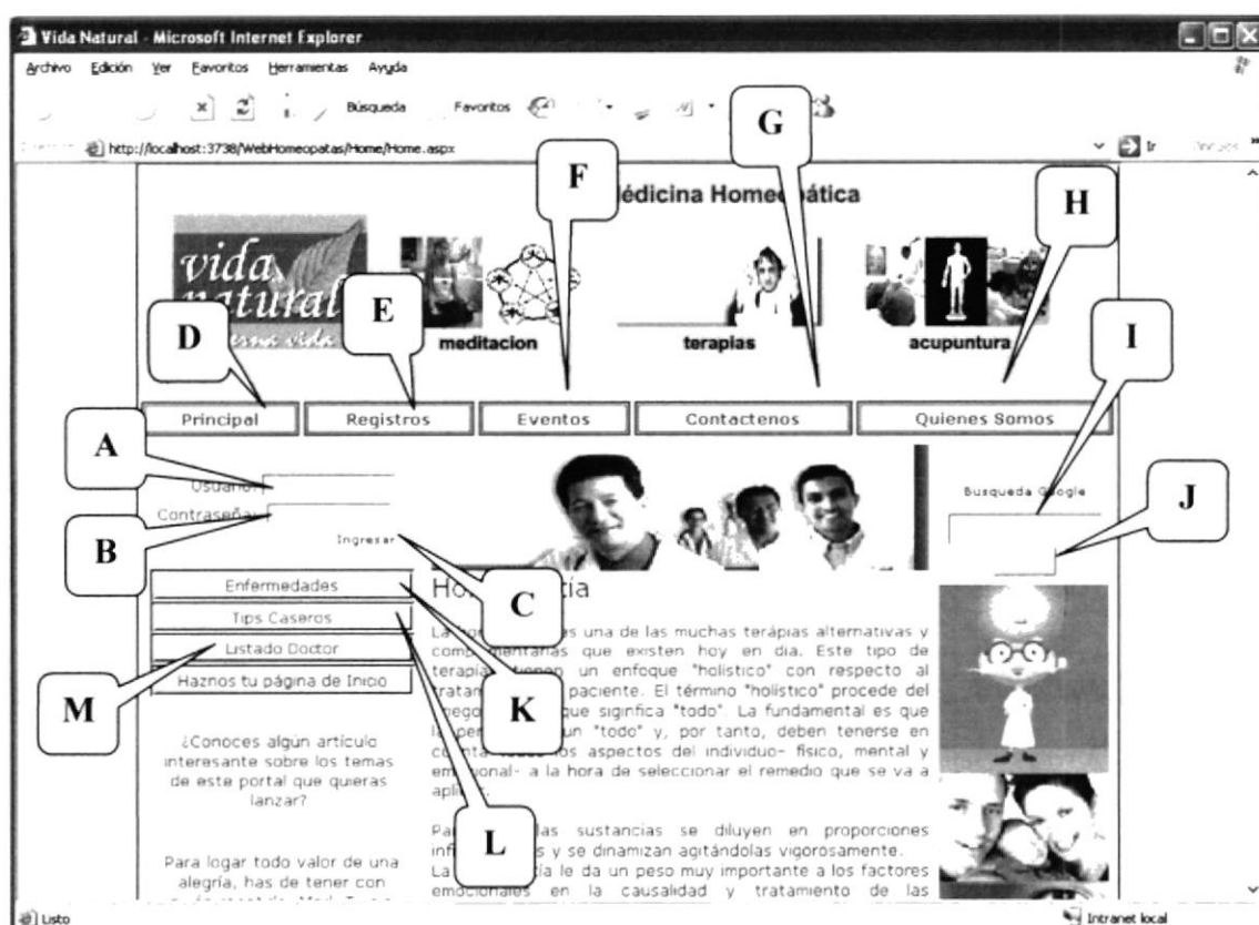
Figura 21. Página principal
