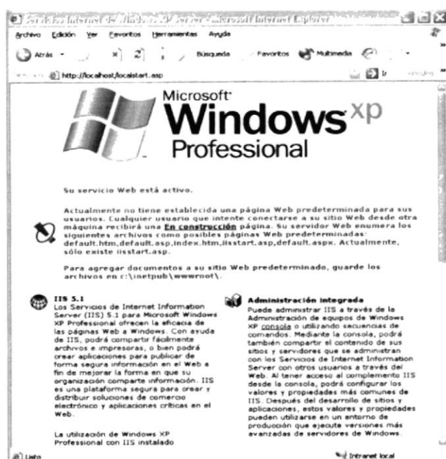
Figura 17. LocalHost
