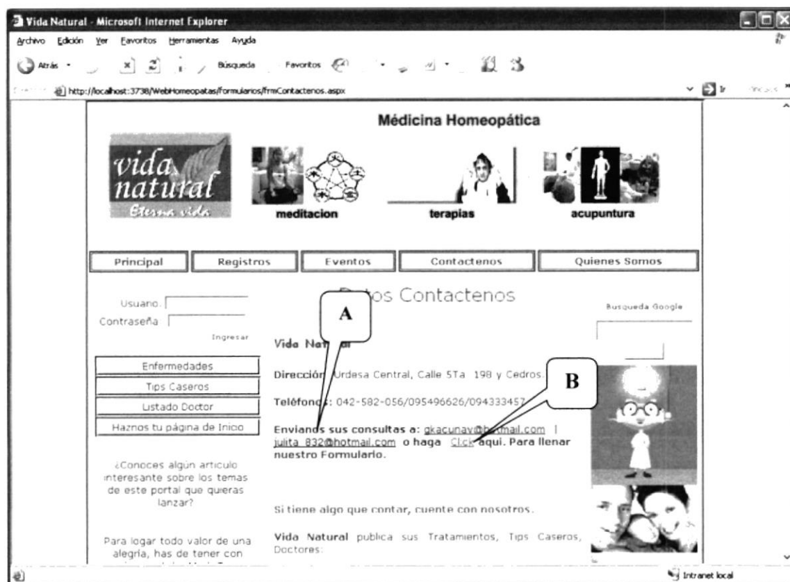
Figura 24. Página Contáctenos
