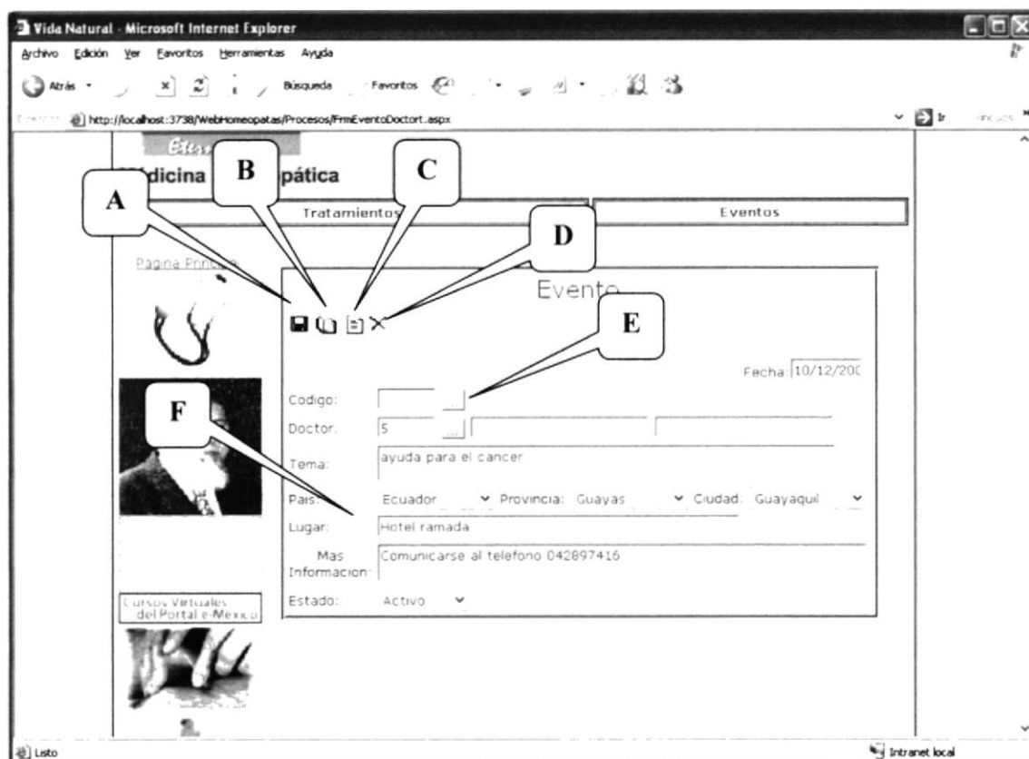
Figura 31. Página Eventos
