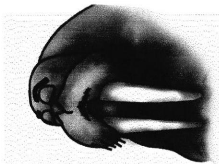
Fig. 9-12 Primer Plano
