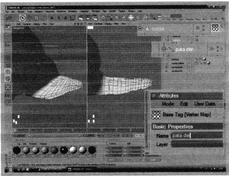
Fig. 9-77: Selección Especial
