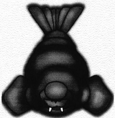
Fig. 9-10: Arriba
