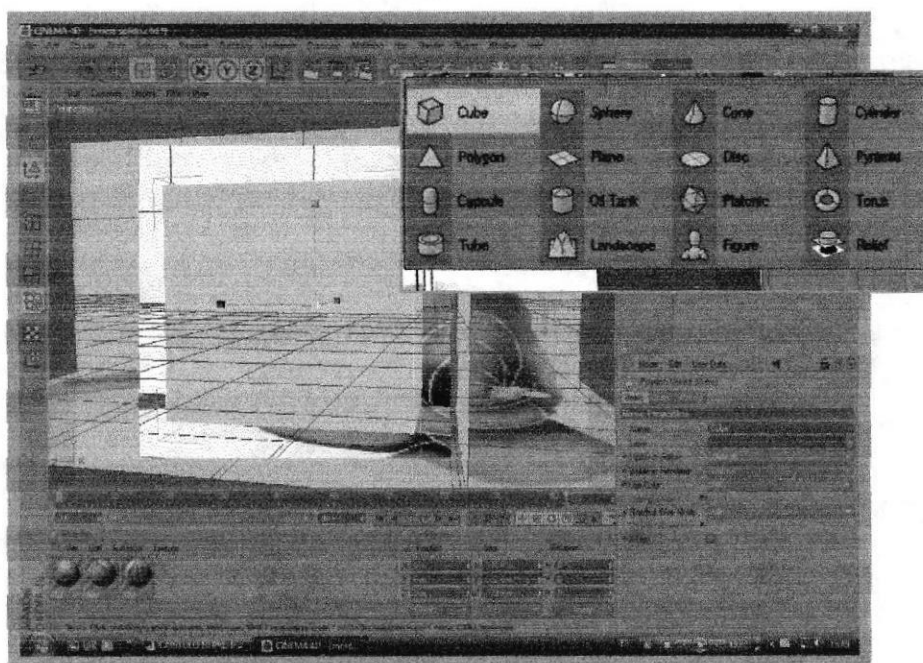
Fig. 9-22: Objeto Primitivo
