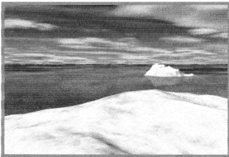
Fig. 9-65: Escenario Final
