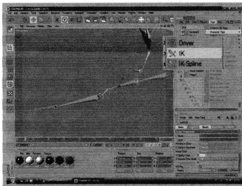
Fig. 9-93: Tag IK
