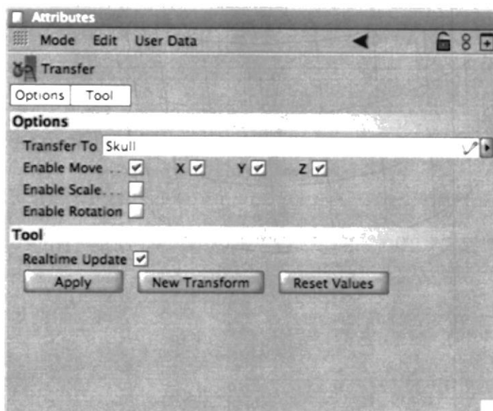
Figura 6-56: Ventana de atributos de Transfer
