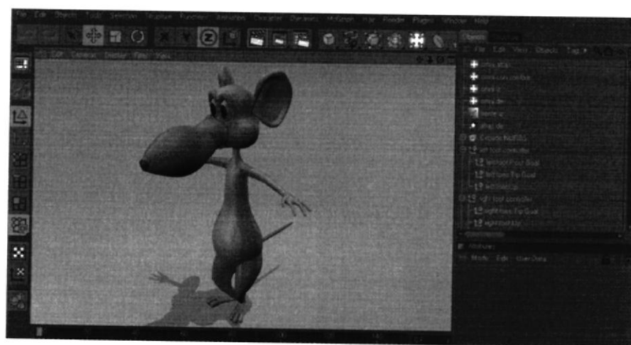
Figura 6-27: Quinta Luz.
