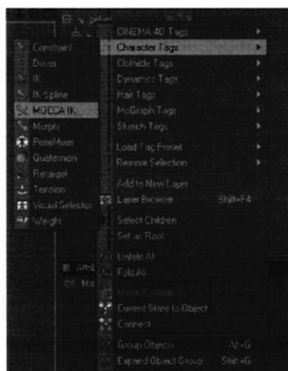
Figura 6-45: MOCCA IK
