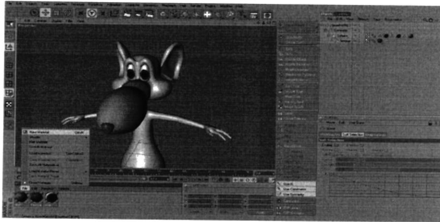
Figura 6-28: Aplicando texturas.
