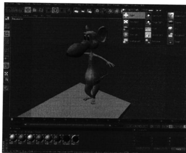
Figura 6-26: Cuarta Luz.
