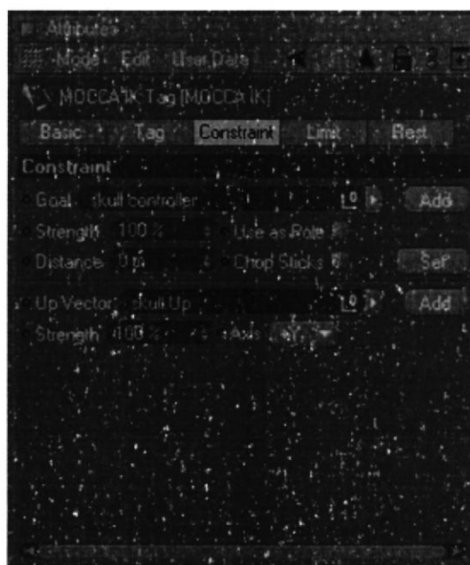
Figura 6-62: Strenght 100%.
