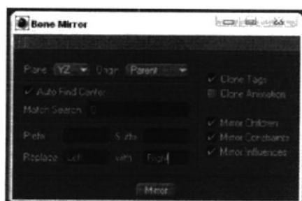
Figura 6-54: Bone Mirror.
