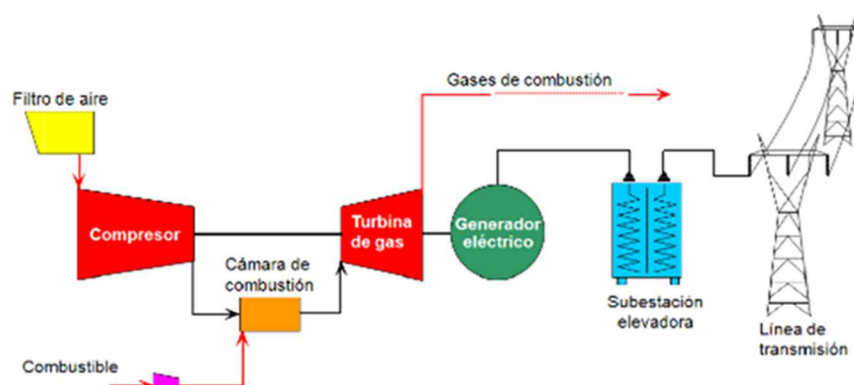
Figura. 2.1 Central Turbogás [16]
