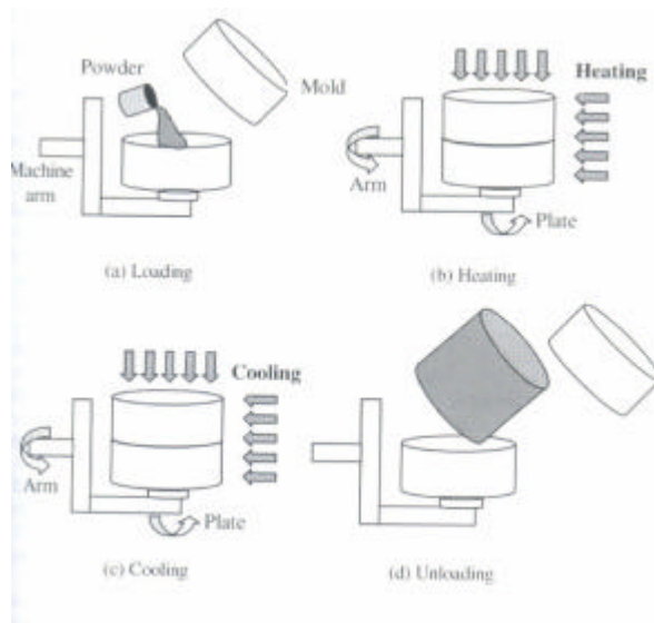
FIGURA 2.10 ESQUEMA DEL PROCESO DEL ROTOMOLDEO. SACADO DE ROTACIONAL MOLDING: A PRACTICAL GUIDE DE PAUL NUGENT
