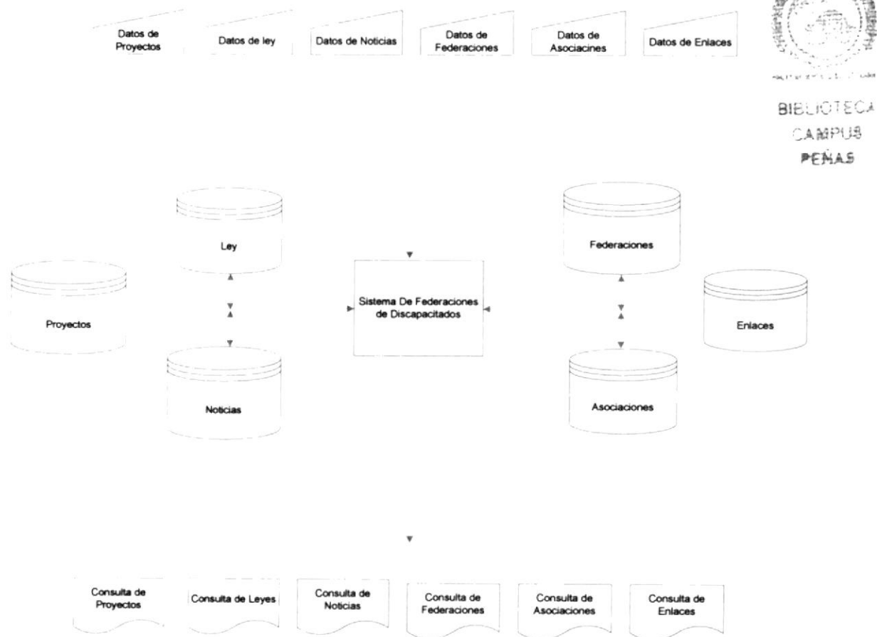
Figura 4.1. Diagrama General del Sitio Web
