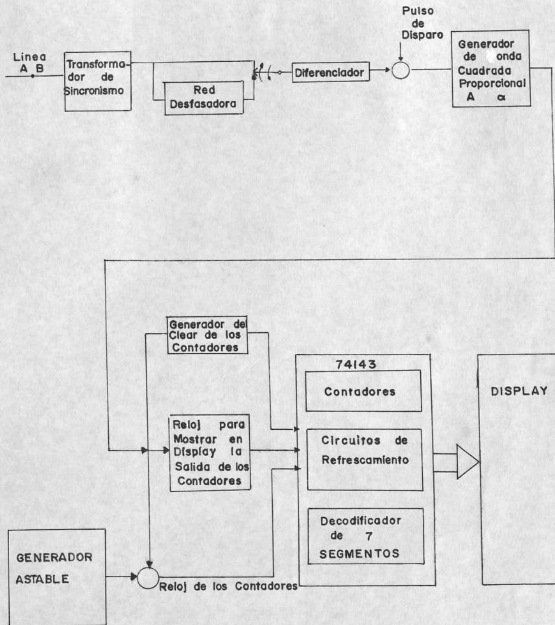
6.1 Diagrama de Bloques del Circuito.
