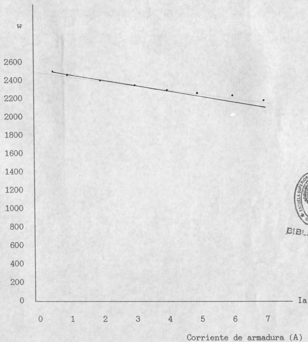
Figura # 7.16.- Gráfico de velocidad ( w ) versus corriente de armadura ( I_a ), Lazo abierto, conducción continua.
