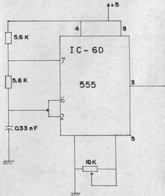
Figura # 6.4.- Generador Astable.
