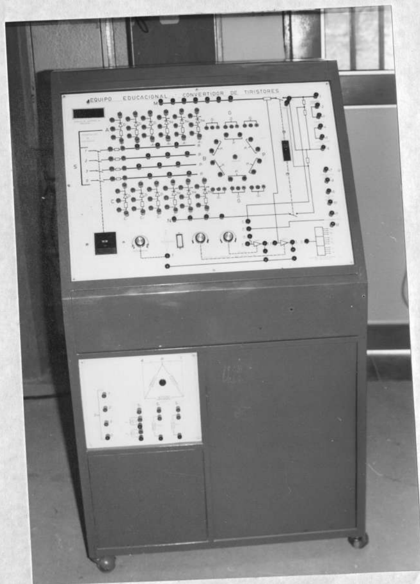
Figura # 1.1.- Vista Frontal del Equipo
