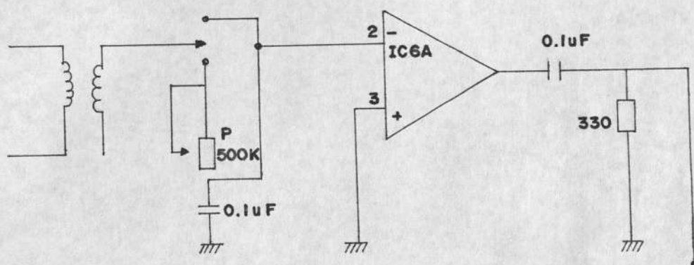
Figura # 6.2.- Red desfasadora y diferenciadora
