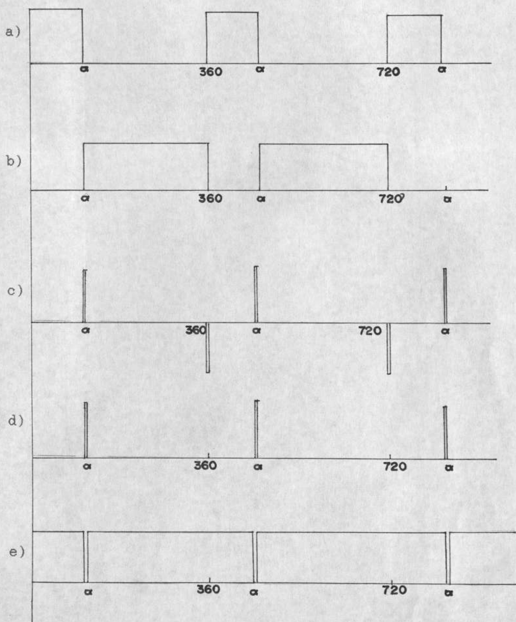
Figura # 6.8.- Señales para la obtención del reloj del latch.
