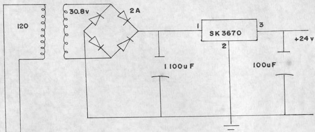
Figura # 2.3.- Fuente de +24 VDC.
