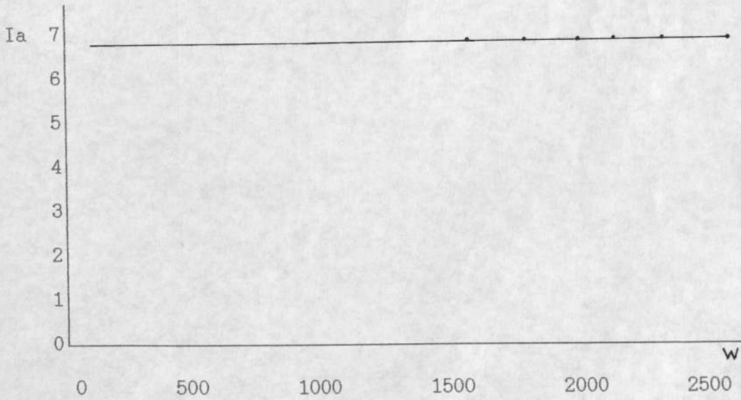
Figura # 7.18 - Corriente de armadura versus velocidad
