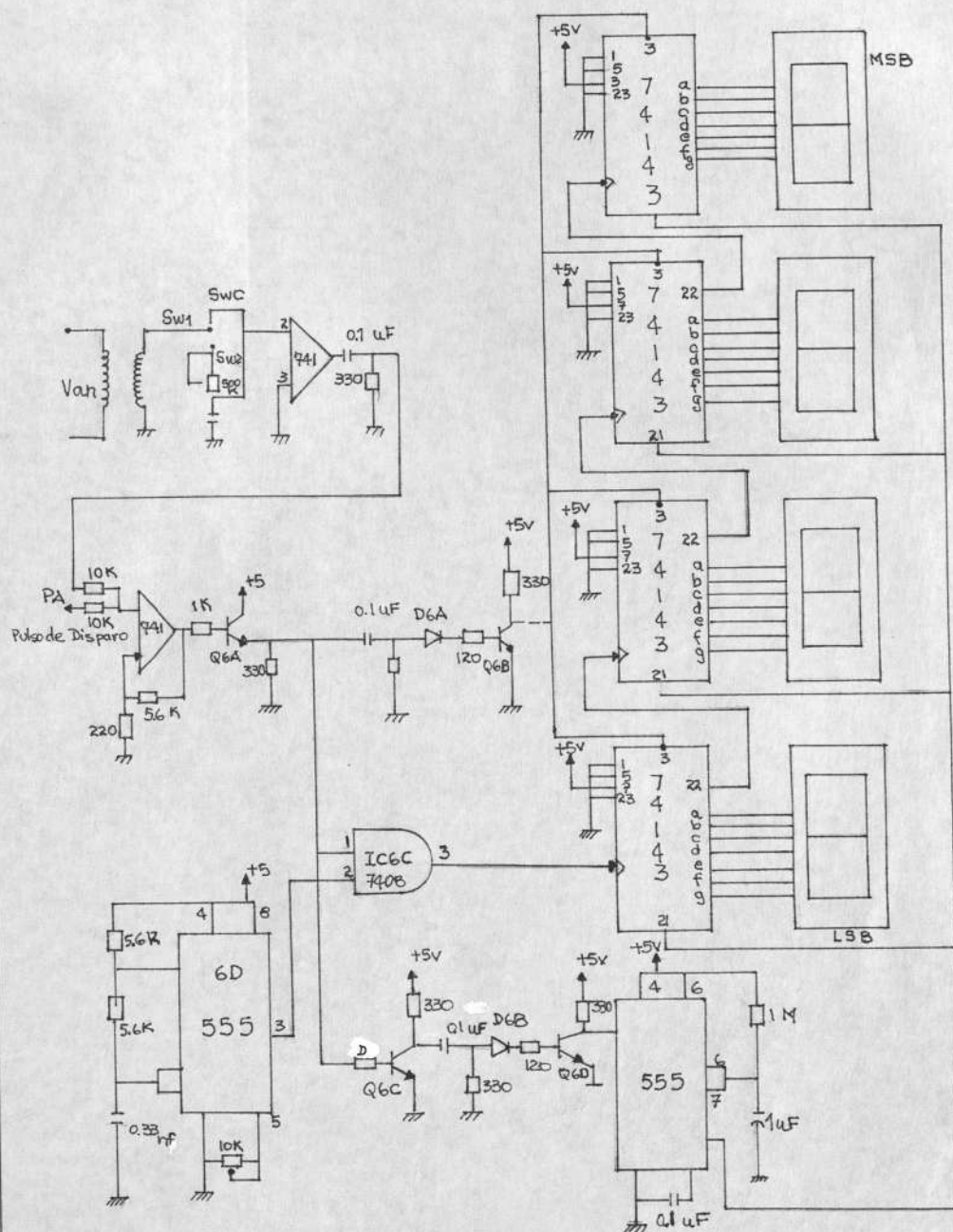
Figura # 6.9.- Circuito del Medidor de Angulo de Disparo.
