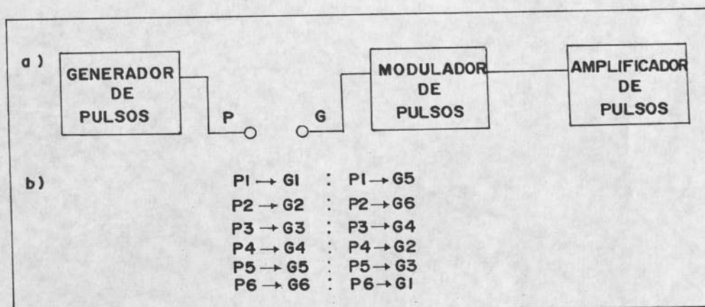
Figura # 3.8.- a) Localización de los terminales P y G. b) Conexiones necesarias para secuencia de la figura # 3.6.
