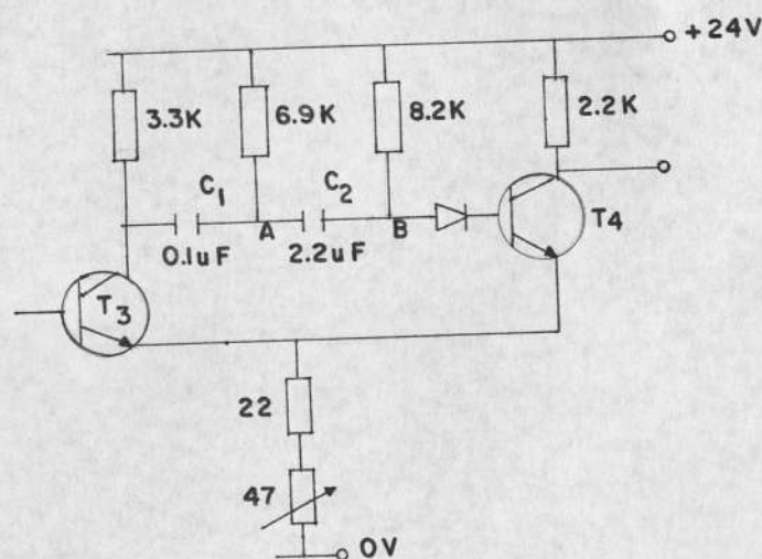
Figura # 3.4 .- Comparador y Generador de Pulsos.
