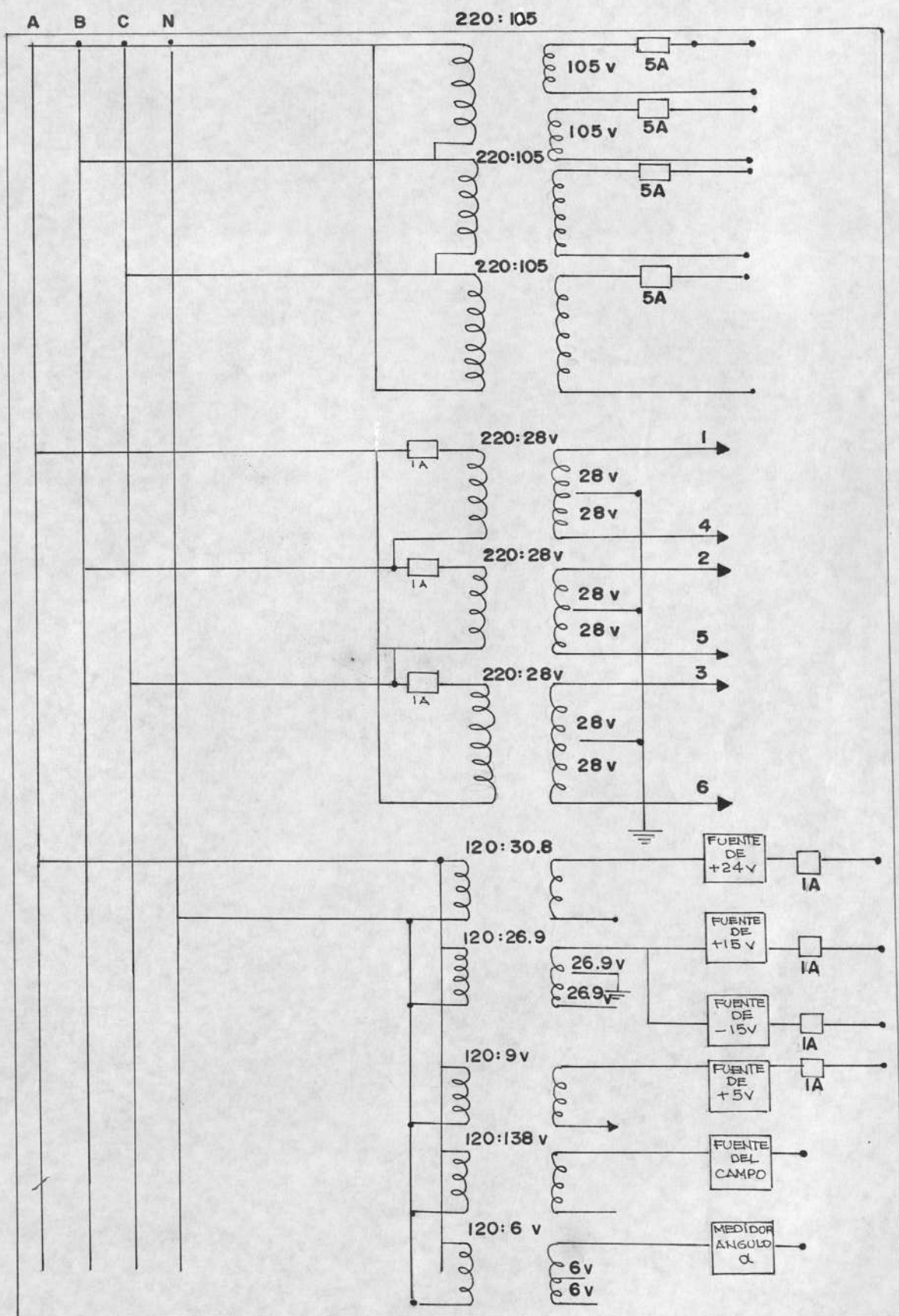
Figura # 2.1.- Diagrama de Transformadores y Fusibles
