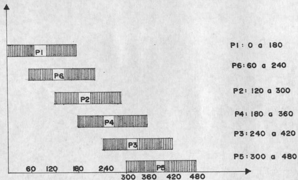
Figura # 3.5.- Rango de acción de los 6 pulsos de Disparo
