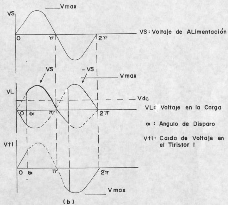
Figura # 4.2.- Rectificación Monofásica de Onda Completa.
