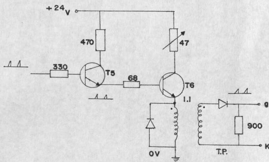
Figura # 3.11.- Circuito Amplificador de Pulsos.
