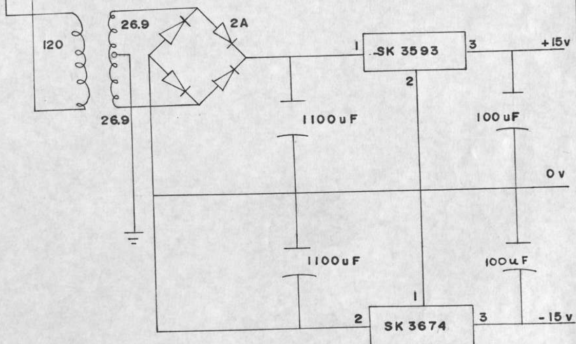
Figura # 2.4.- Fuente de +15 V y -15 V.
