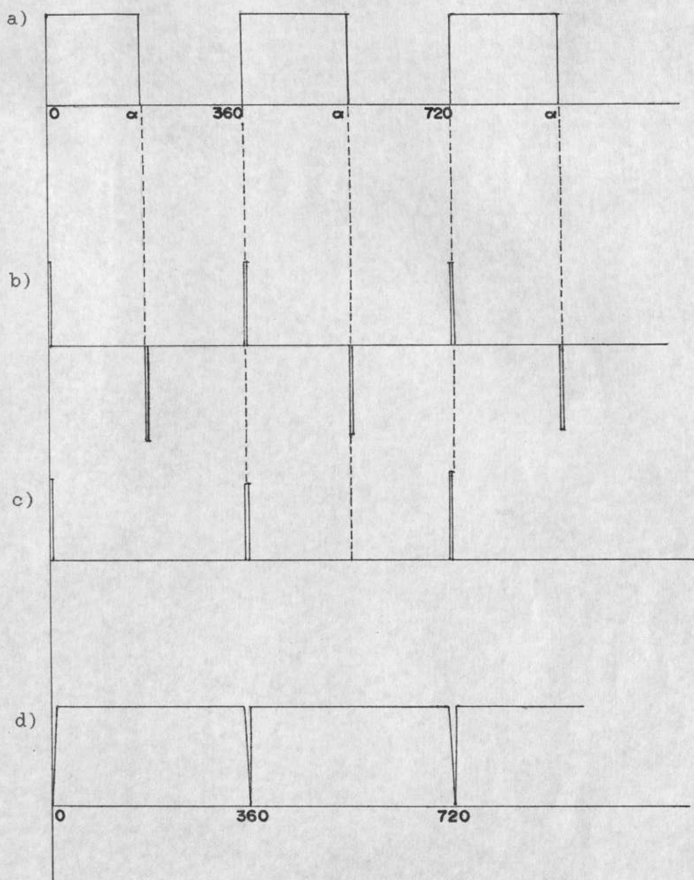
Figura # 6.6.- Señales para la obtención del Clear de los Contadores.
