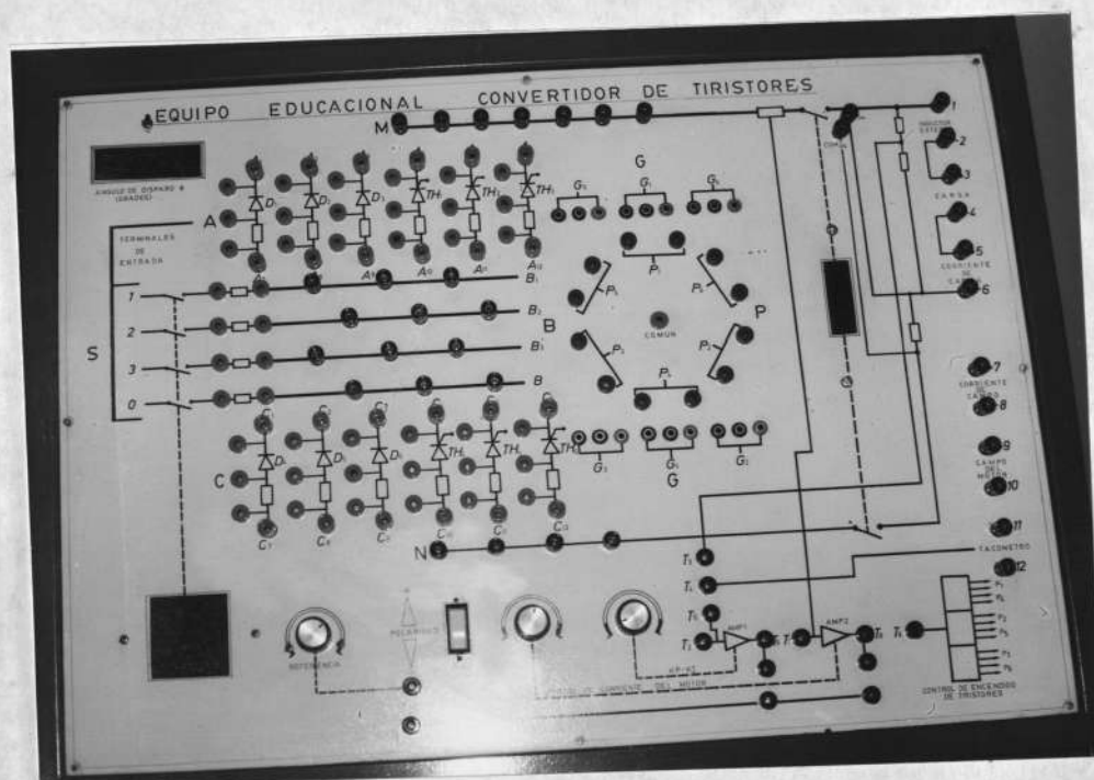
Figura # 1.2 .- Vista Frontal Superior.
