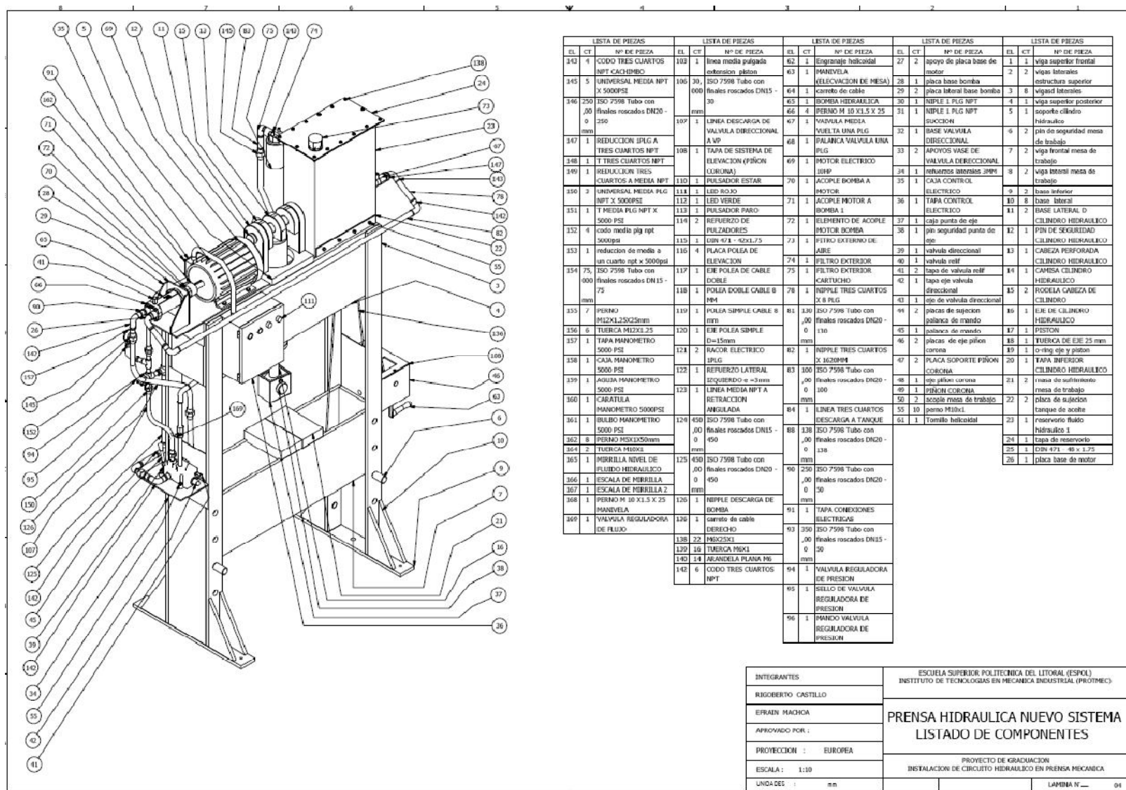
Acoplamiento de sistema hidráulico a prensa mecánica
