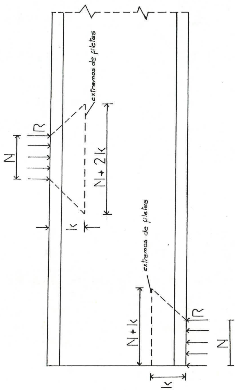
FIGURA N°7 Aplastamiento del alma de una Viga
