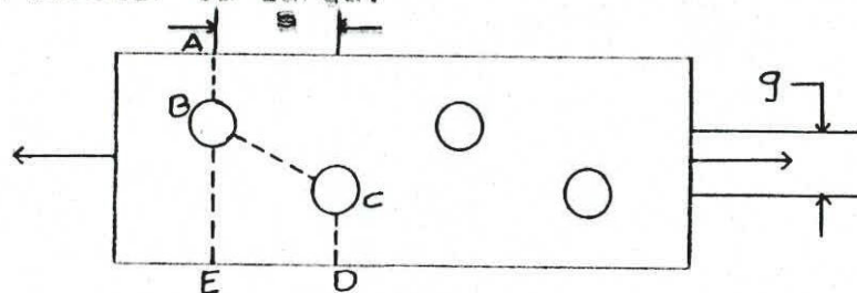
Figura No. 1 AGUJEROS ALTERNADOS
