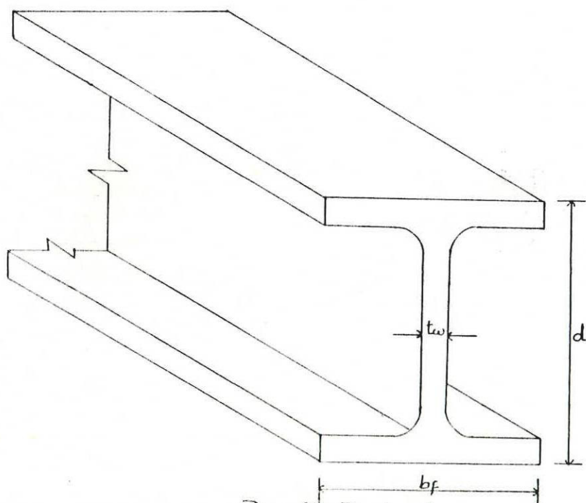
Perfil Rolado
