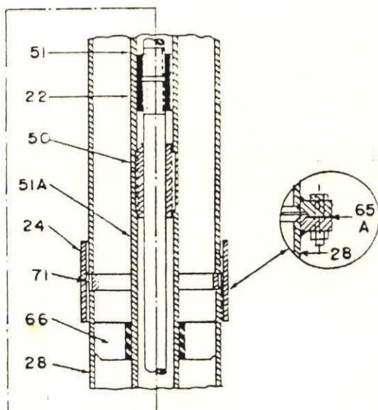
Fig. 12 — Bomba de construção reclinada com descarga subterrânea. (Lubrificação à água)
