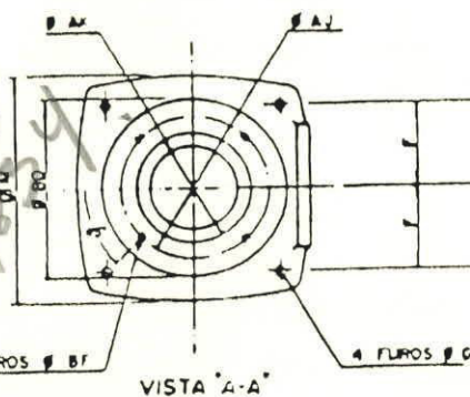
VISTA "A-A"
