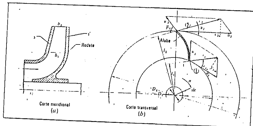
Fig # 1.5 Sección media de un rodete
