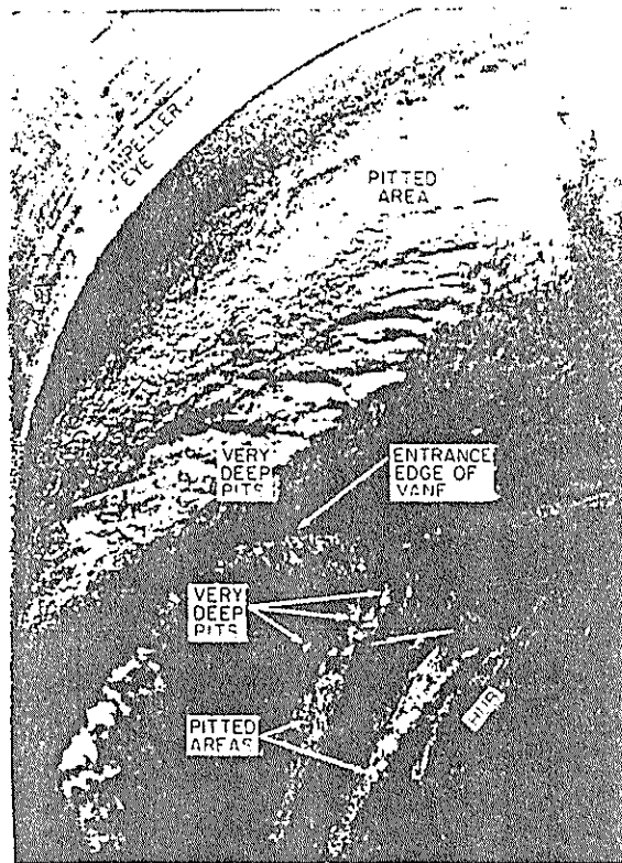
Fig. # 4.1 Impeller con cavilación
