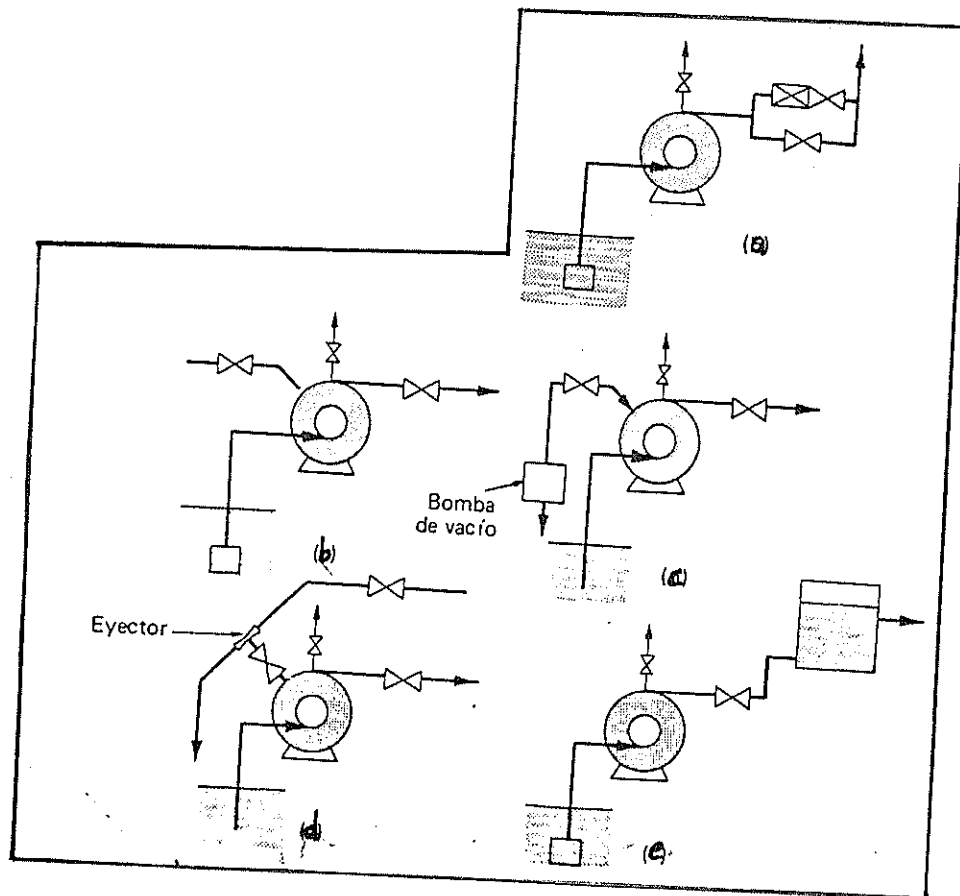
Fig. # 2.3 Tipos de cebado
