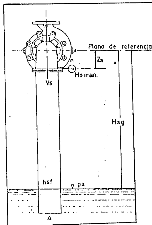
Fig # 3.1 Parámetros del NPSH
