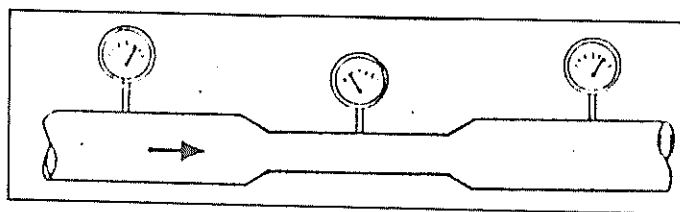
Fig. 1.1 Flujo en un conducto
