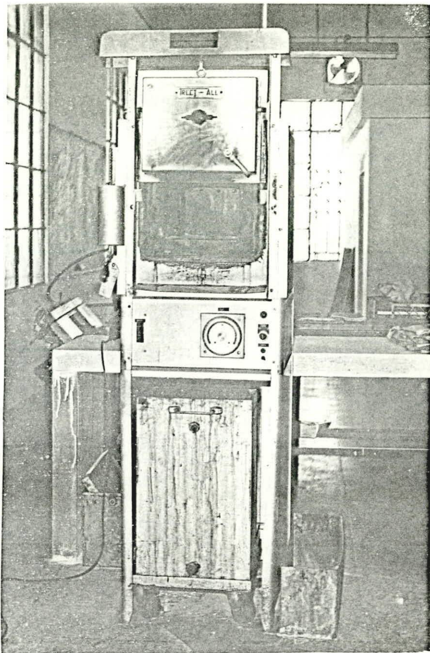
HORNO EXPERIMENTAL DE LIMBERG DE MUFLA DE HASTA 1.100°C CON CONTROL AUTOMATICO DE TEMPERATURA CON TOLERANCIA DE \pm 5^{\circ}\text{C}
