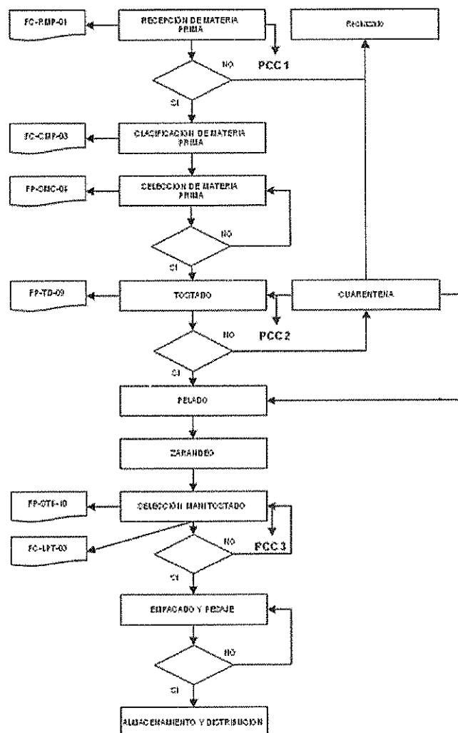
Figura 1.3: Diagrama de Flujo de Elaboración de maní tostado
