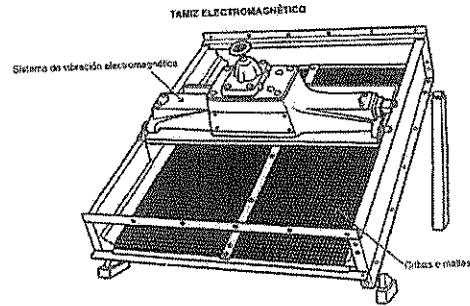
Figura 4.2: Zaranda Vibratoria
