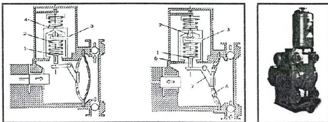
FIGURA 2.6: BOMBAS DE DOBLE DIAFRAGMA HIDRÁULICAS
