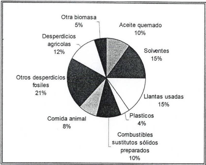
FIGURA 1.3: TIPOS DE DESECHOS USADOS COMO COMBUSTIBLES ALTERNATIVOS A NIVEL MUNDIAL FUENTE: AFR Score L2 – 12.04
