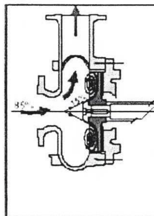
FIGURA 2.2: BOMBA CENTRIFUGA, DISEÑO PARA POZO SECO
