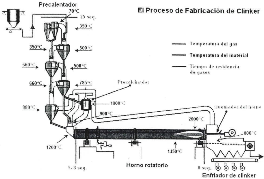
FIGURA 1.2: PROCESO DE FABRICACIÓN DEL CLINKER
