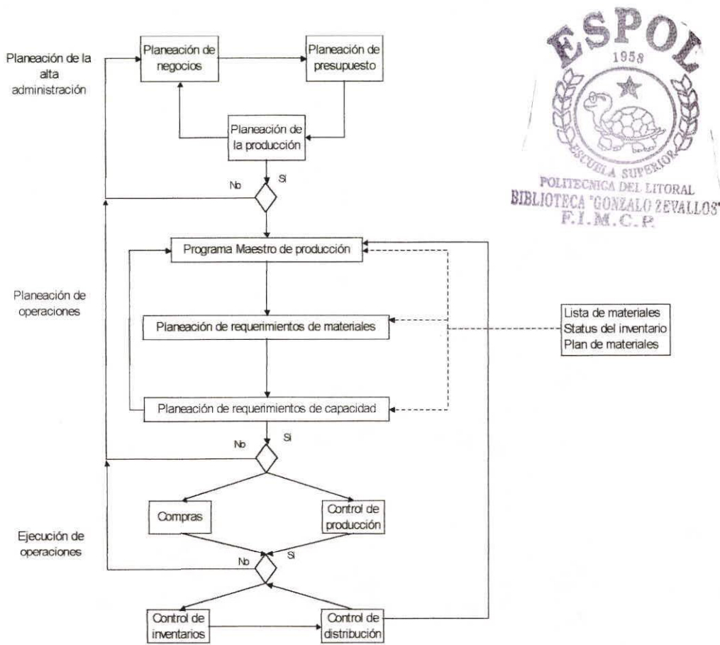
Figura 2.11 Sistema Básico del MRP II
