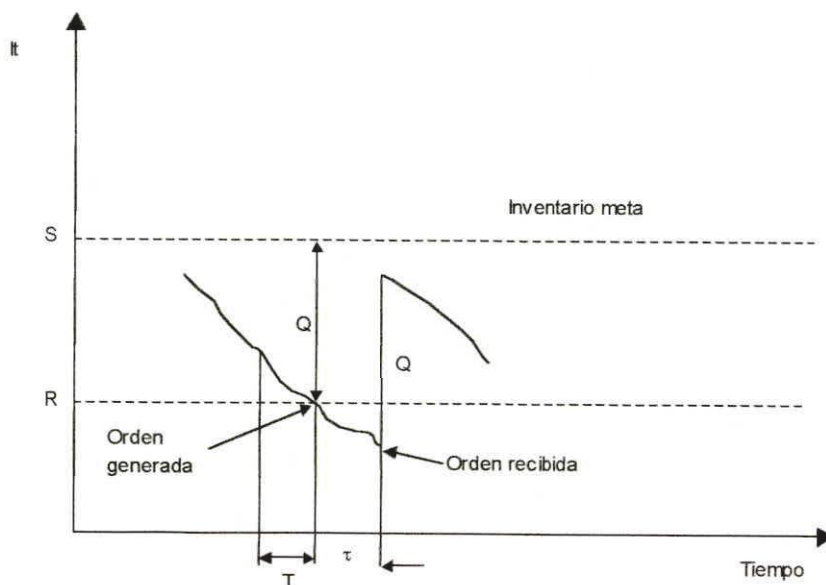
Figura 2.6 Método Periódico
