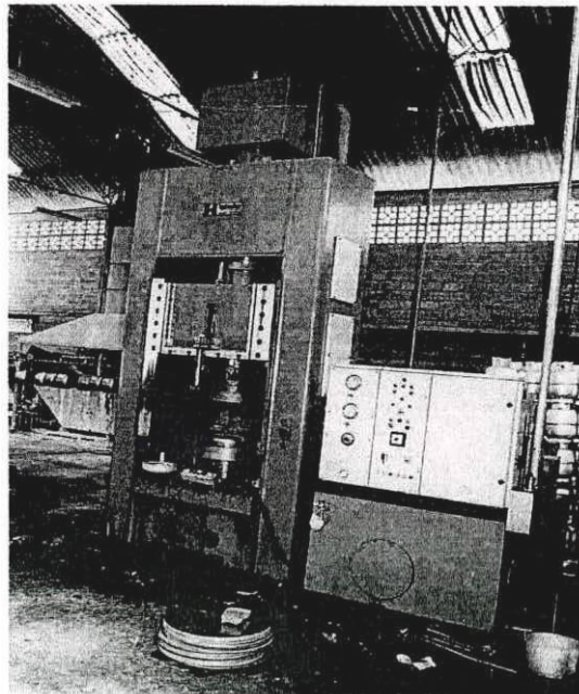
FIGURA 1.12 PRENSA HIDRAÚLICA
