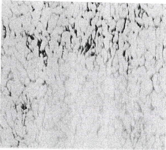
FIGURA 2.3 MICROESTRUCTURA DE DISCO DE ALUMINIO
