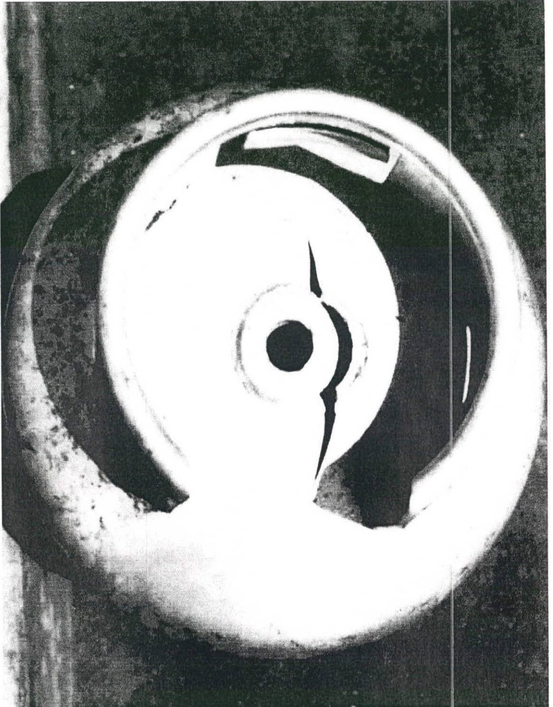
FIGURA 1.11 FALLA DE SOLDADURA DE PORTA VALVULA
