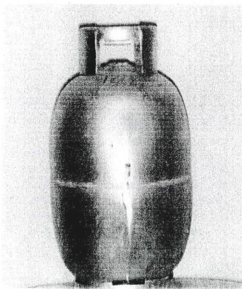
FIGURA 2.11 PRUEBAS DE ROTURA DE CILINDRO DE ALUMINIO
