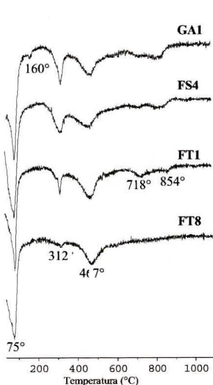
Figura 4.5- Curvas termogravimétricas da fração argila das quatro amostras selecionadas, após a aplicação do método DCB.
