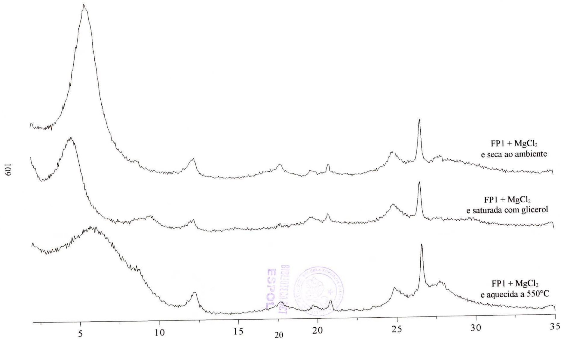
Anexo 10- Difratomogramas da fração argila da amostra FP1 saturada com \text{MgCl}_2 : seca ao ambiente, saturada com glicerol e, aquecida a 550^\circ\text{C} .
