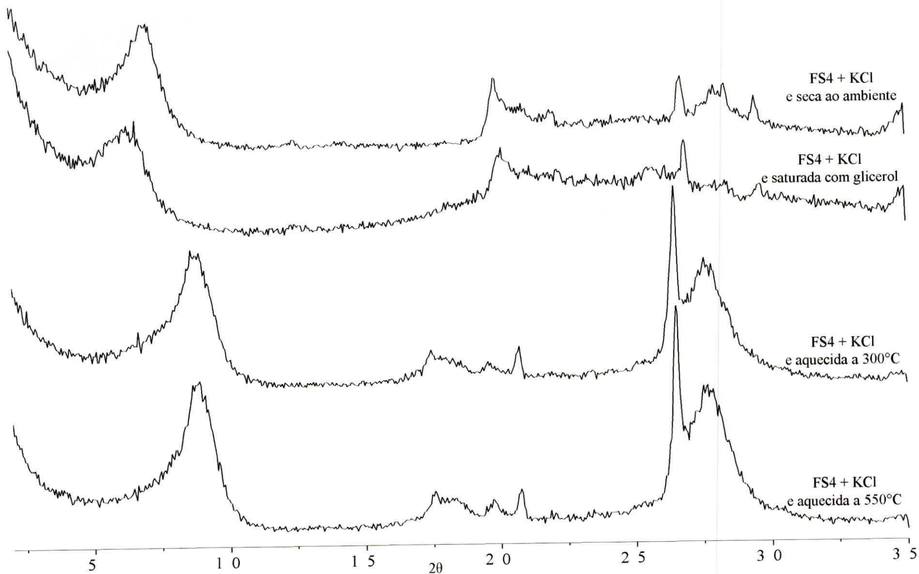
Anexo 07- Difrátogramas da fração argila da amostra FS4 saturada com KCl: seca ao ambiente, saturada com glicerol, aquecida a 350°C e, aquecida a 550°C.
