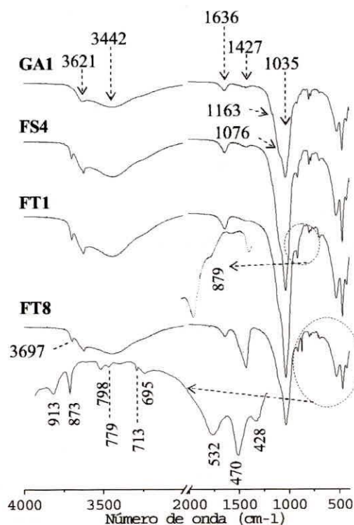
Figura 4.6- Espectros do infravermelho da fração argila das quatro amostras selecionadas.
