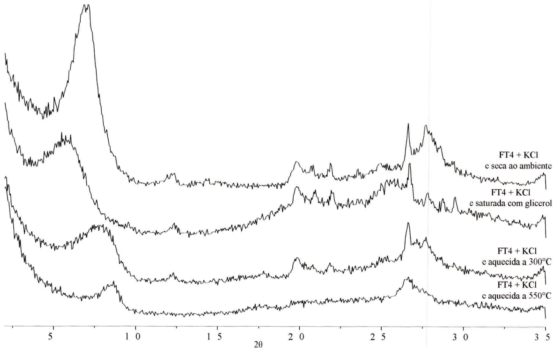
Anexo 19- Difrátogramas da fração argila da amostra FT4 saturada com KCl: seca ao ambiente, saturada com glicerol e, aquecida a 550^\circ\text{C} .
