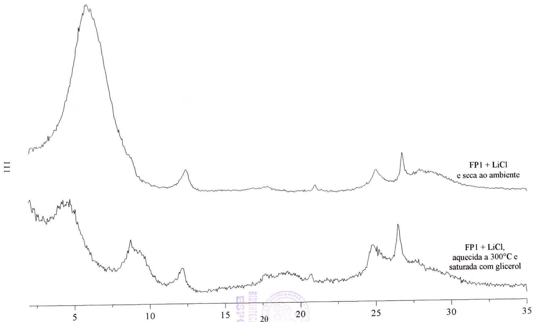
Anexo 12- Difrátogramas da fração argila da amostra FP1 saturada com LiCl: seca ao ambiente e, saturada com glicerol após aquecida a 300°C.
