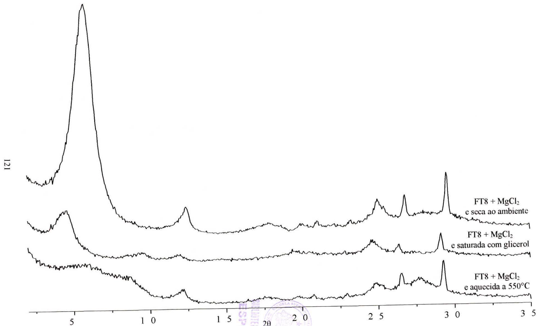
Anexo 22- Difratomogramas da fração argila da amostra FT8 saturada com MgCl 2 : seca ao ambiente, saturada com glicerol e, aquecida a 550°C
