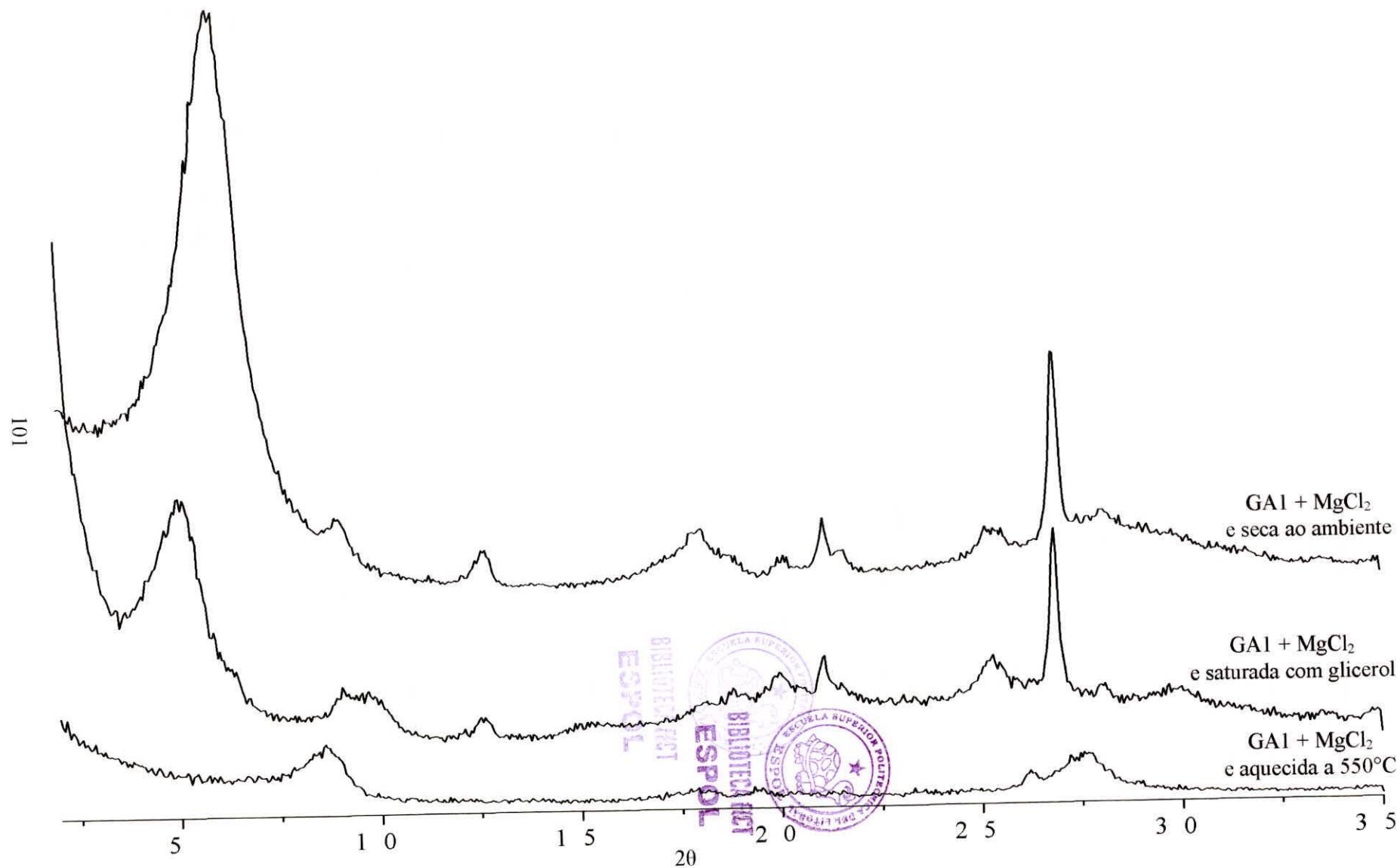
Anexo 02- Difratomogramas da fração argila da amostra GA1 saturada com MgCl 2 : seca ao ambiente, saturada com glicerol e, aquecida a 550°C
