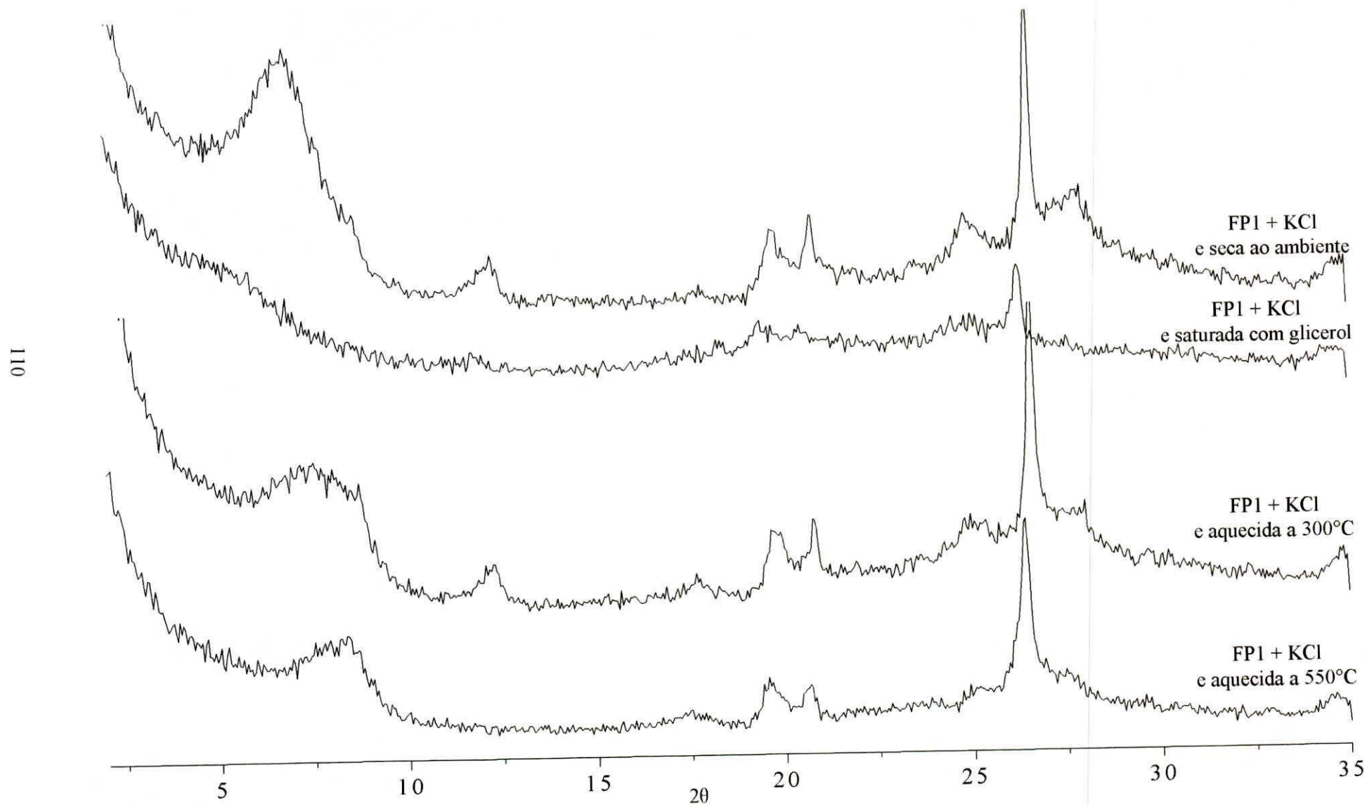
Anexo 11- Difratomogramas da fração argila da amostra FP1 saturada com KCl: seca ao ambiente, saturada com glicerol, aquecida a 350°C e, aquecida a 550°C.
