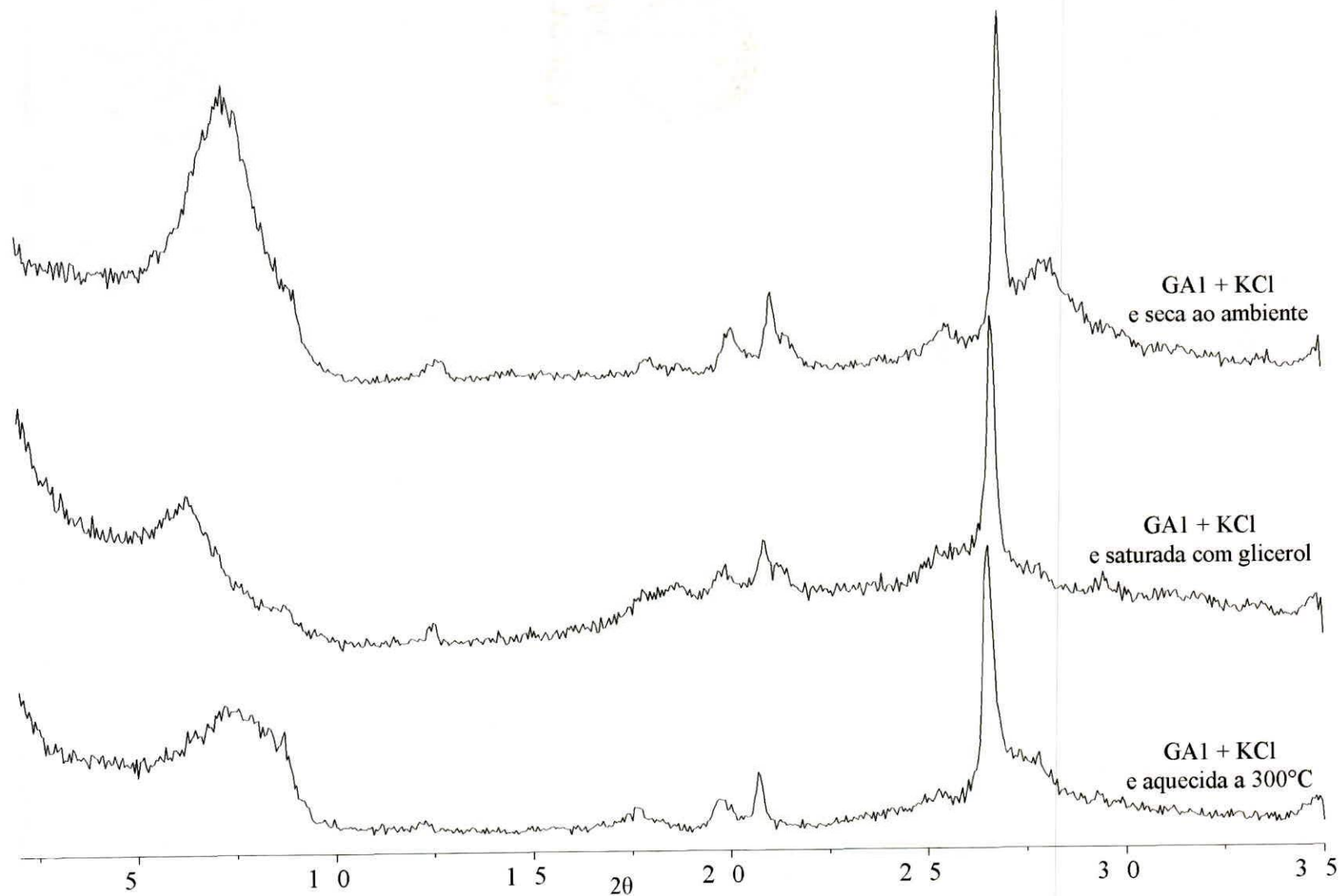
Anexo 03- Difractogramas da fração argila da amostra GA1 saturada com KCl: seca ao ambiente, saturada com glicerol e, aquecida a 550°C.
