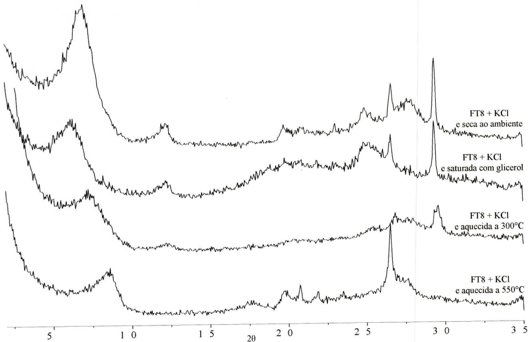
Anexo 23- Difrátogramas da fração argila da amostra FT8 saturada com KCl: seca ao ambiente, saturada com glicerol e, aquecida a 550^\circ\text{C} .
