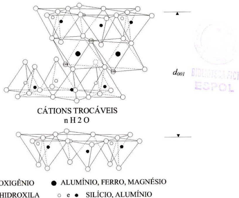
Figura 3.3- Estrutura cristalina da montmorilonita (Grim 1962)
