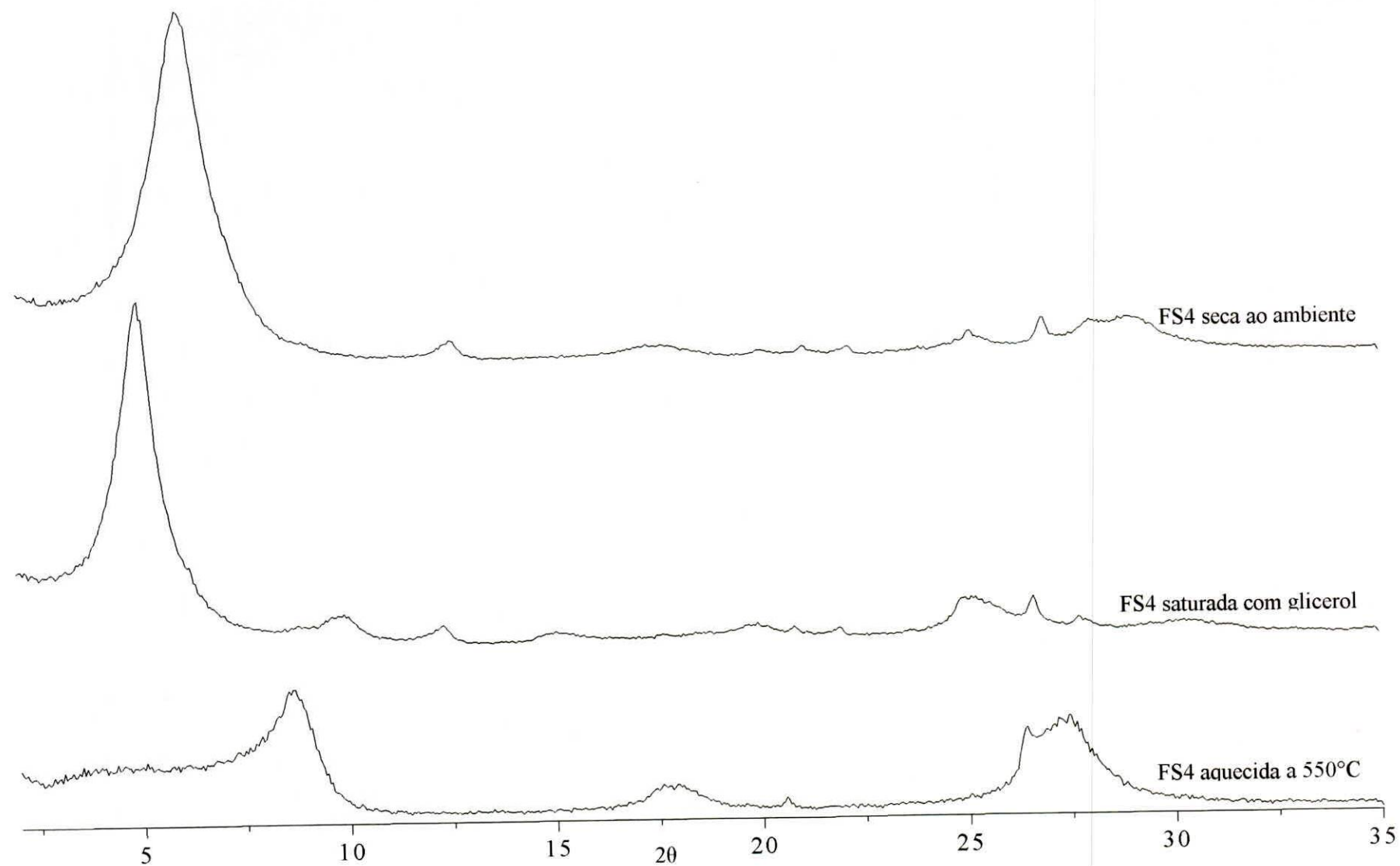
Anexo 05- Difratogramas da fração argila da amostra FS4 seca ao ambiente, saturada com glicerol e, aquecida a 550°C.
