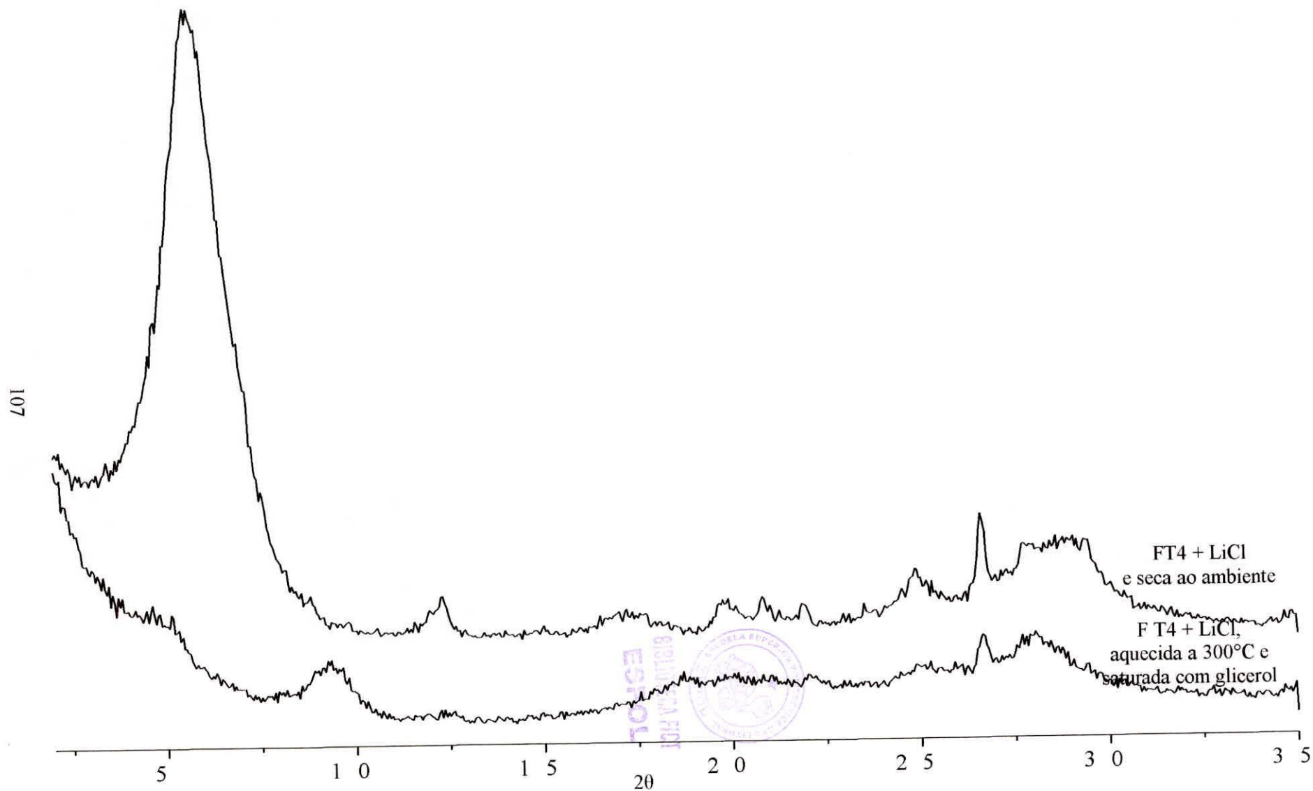
Anexo 08- Difratogramas da fração argila da amostra FS4 saturada com LiCl: seca ao ambiente e, saturada com glicerol após aquecida a 300°C.
