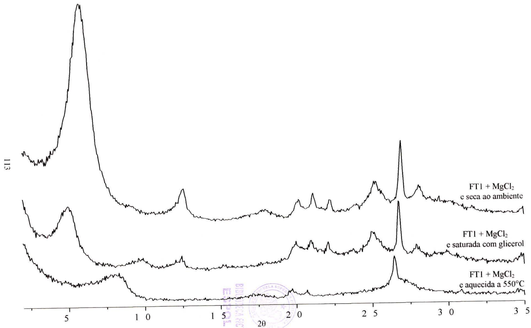
Anexo 14- Difratomogramas da fração argila da amostra FT1 saturada com MgCl 2 : seca ao ambiente, saturada com glicerol e, aquecida a 550°C.
