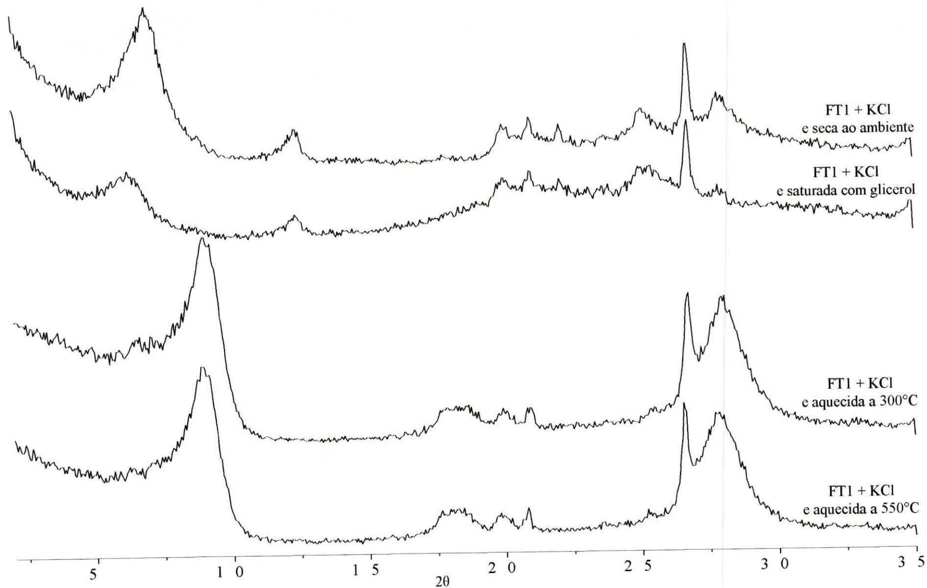
Anexo 15- Difratogramas da fração argila da amostra FT1 saturada com KCl: seca ao ambiente, saturada com glicerol, aquecida a 350^\circ\text{C} e, aquecida a 550^\circ\text{C} .
