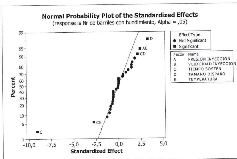
Figura 4.4. Efectos del proceso a analizar
