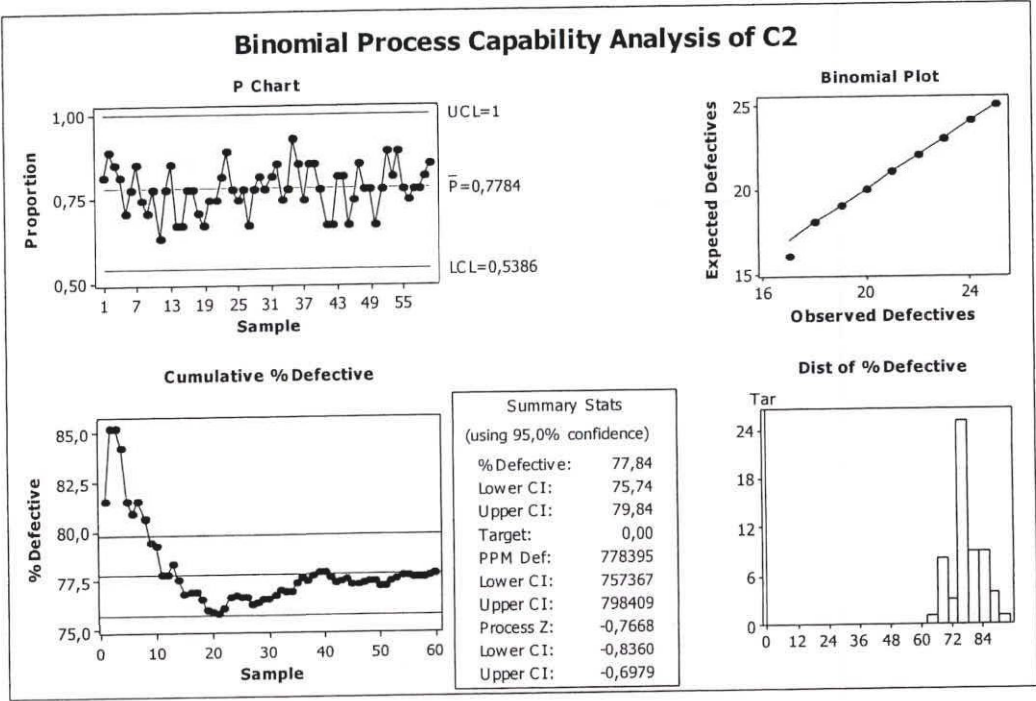
Figura 3.2. Análisis de capacidad por atributo
