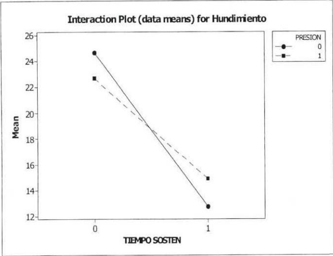
Figura 4.8. Gráfica Presión de inyección *Tiempo sostén
