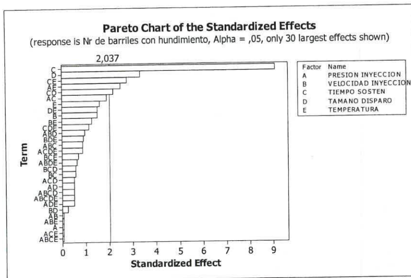
Figura 4.3. Diagrama Pareto de factores involucrados
