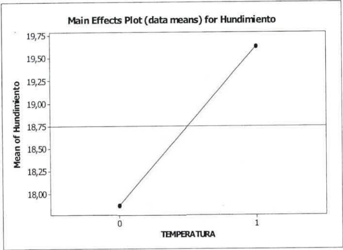
Figura 4.7. Gráfica Temperatura
