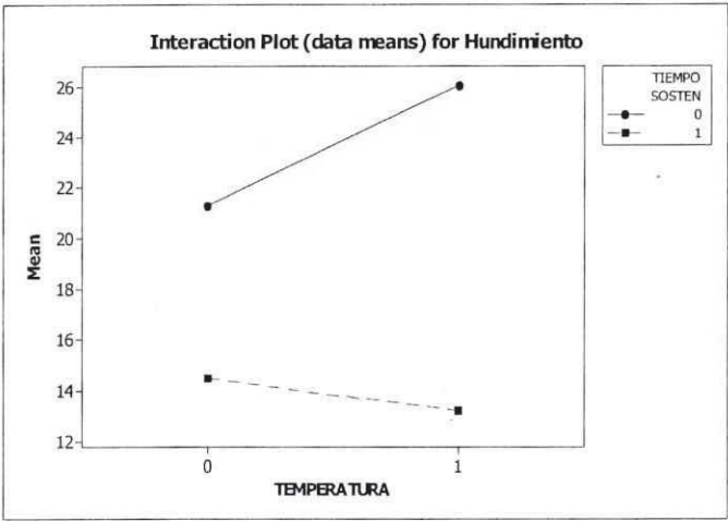
Figura 4.11. Gráfica Tiempo de sostén* Temperatura
