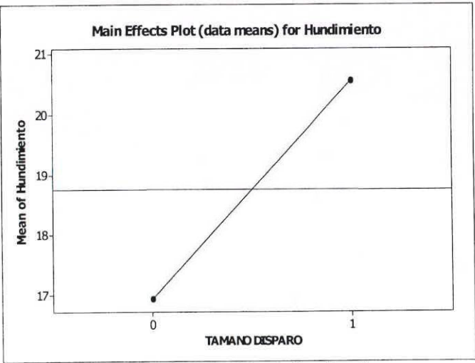
Figura 4.6. Gráfica Tamaño de disparo
