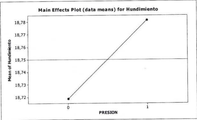
Figura 4.5. Gráfica Presión de inyección
