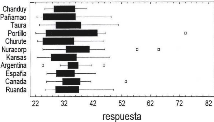
Figura 3.2. Gráfica de Caja y Bigotes del Análisis de los Datos de Residuales mg/kg de Camarón que Llega a la Planta Elaborado por: Carmen Llerena
