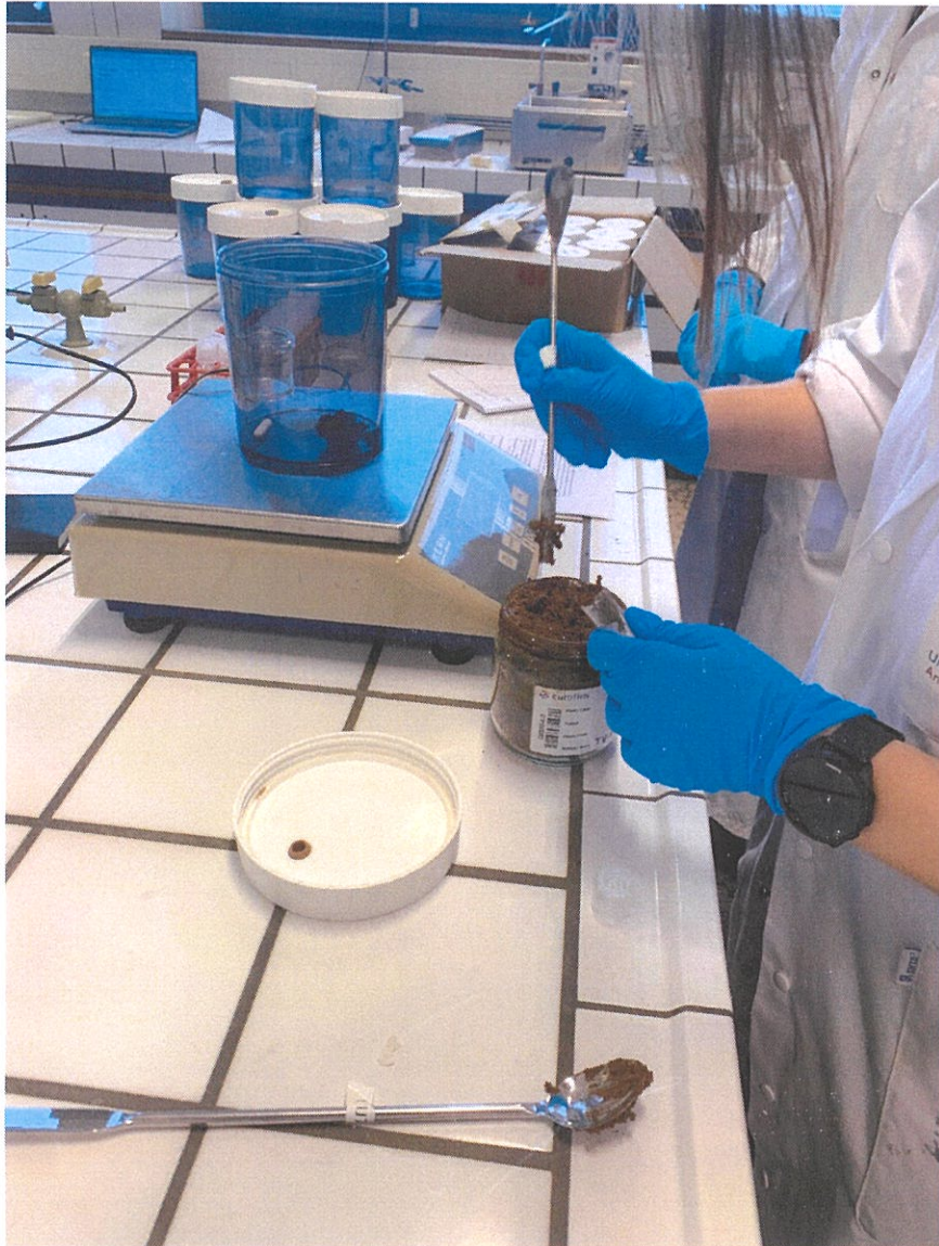
Ilustración 4. Proceso para la determinación de la fracción biodisponible de metales pesados en base a la metodología AVS-SEM.
