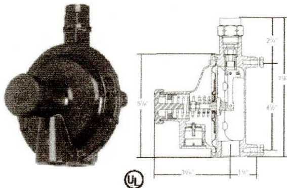
Serie LV4403 SR/TR
