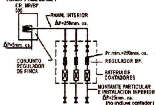
INSTALACION RECEPTORA EN BP. 600mm. ca. CON BATERIA DE CONTADORES; CON REGULADOR DE FINCA Y RED DE MP.
