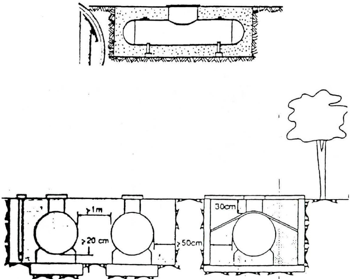
FIGURA 5B. Tanques bajo superficie
