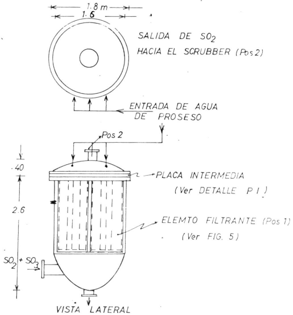
Figura #4 - Lavador Humedo
