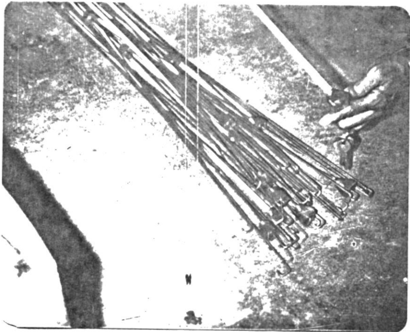
FOTO F11B. Electrodos que conducen la alta tensión de manera concéntrica a los tubos en el interior del precipitador.
