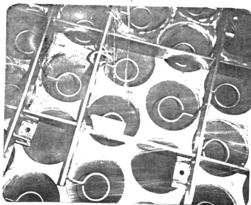
FOTO F10B. Parte interna inferior donde se aprecian los tabos de soporte de los electrodos y con unos conductores que se introducen en los tabos. (Antes del montaje).
