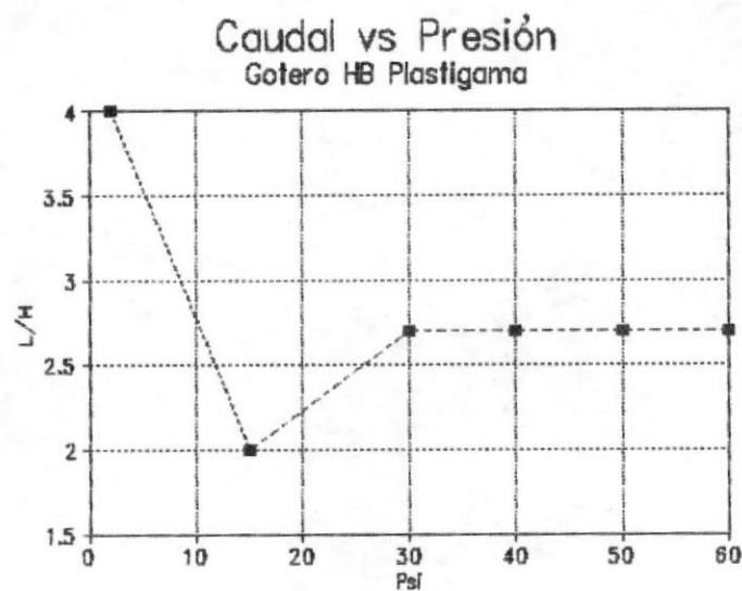
Fig. Nº 1 Curva característica del gotero HB. Ref. 4.
