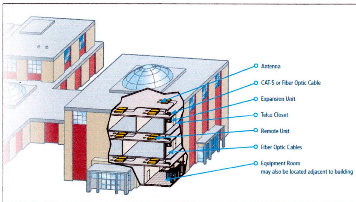
Figura 7 Esquema iDAS
