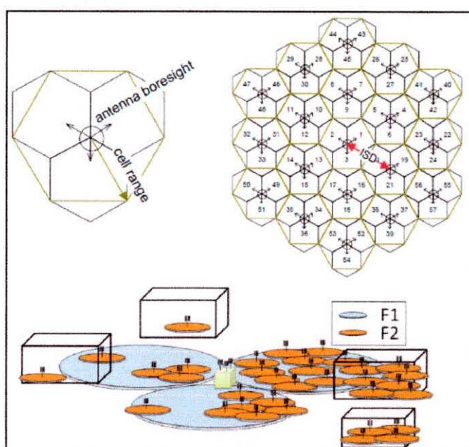
Figura 6 Esquema de red celular
