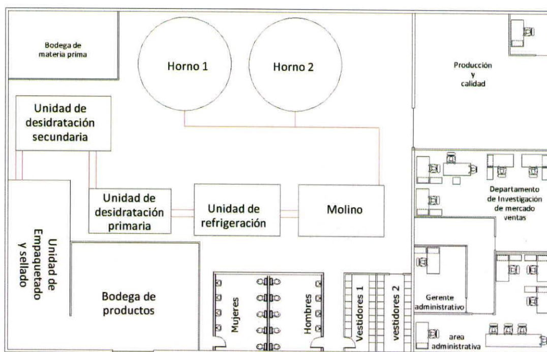
Fig. 20 Plano fabrica La Avanzada
