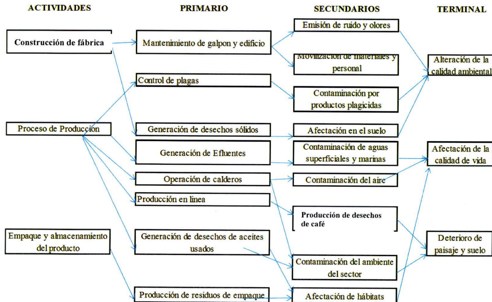
Fig. 23 Diagrama de Redes (Etapa de Construcción 1-2).
