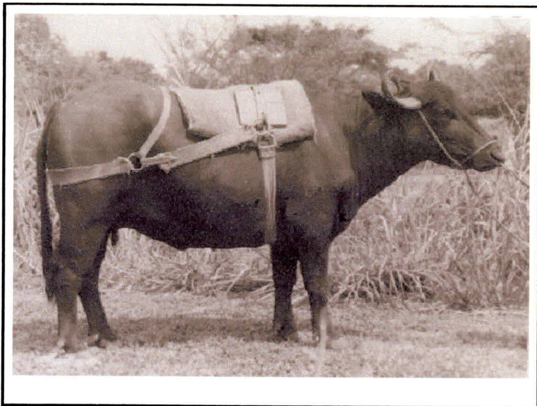
Foto 13. Mediante el retranco se evita que una carreta o la carga transportada se deslice hacia adelante, en especial en terrenos pendientes evitando así accidentes.
