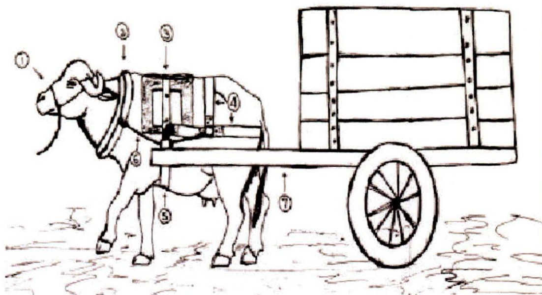
Figura 1. Descripción de aperos. 1) Cabezal. 2) Collera. 3) Galápago. 4) Retranco. 5) Cincha. 6) Cadena. 7) Lanza.
