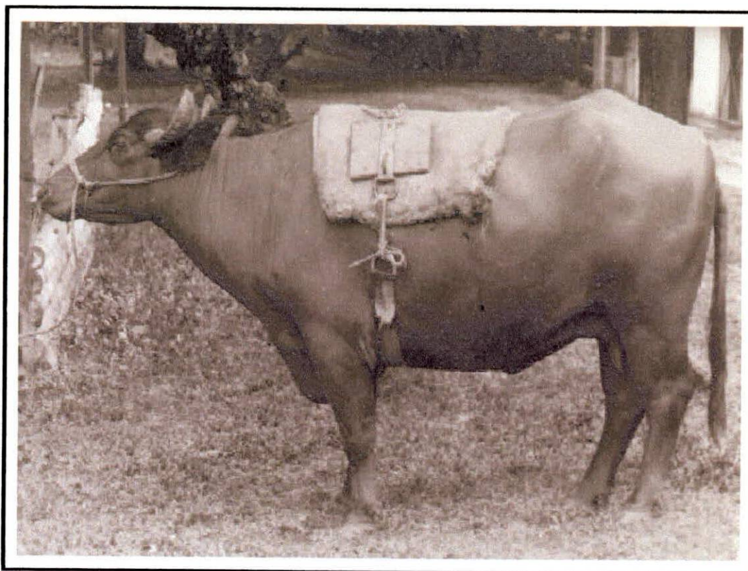
Foto 12. El galápago es el apero que soporta sobre la espalda del búfalo el peso de los implementos que tira o transporta el animal.
