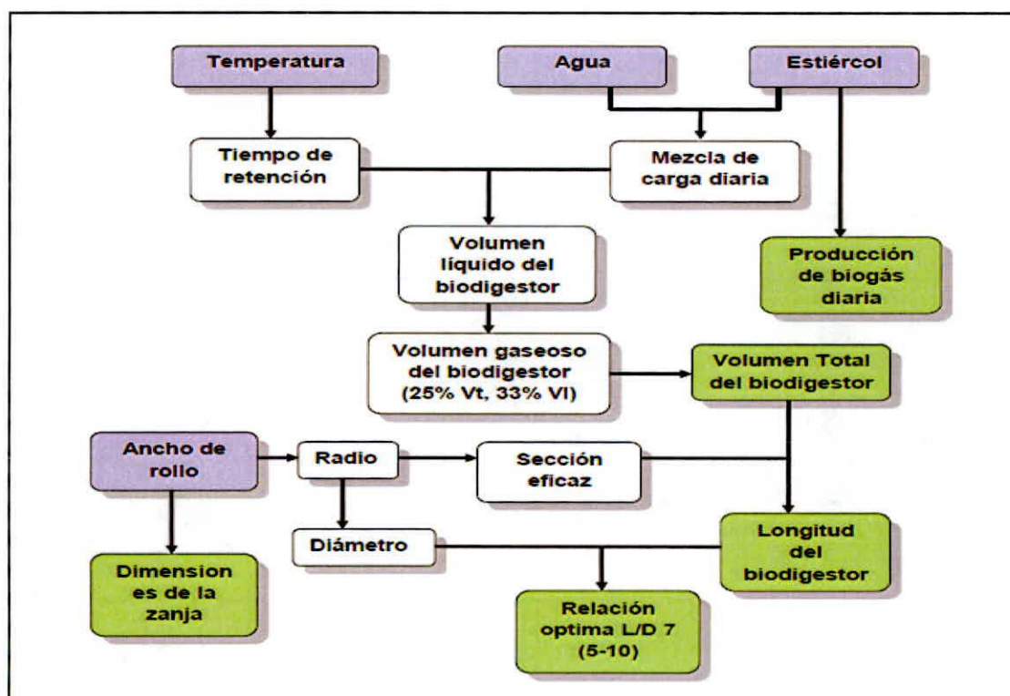
Figura 6.4: Esquema de metodología de diseño de biodigestores Fuente: Guía de diseño y manual de instalación de biodigestores familiares.
