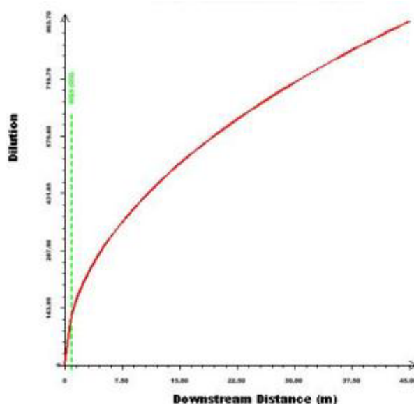
Figura 4.27 CorVue diagrama de dilución vs distancia aguas abajo grilla 50
