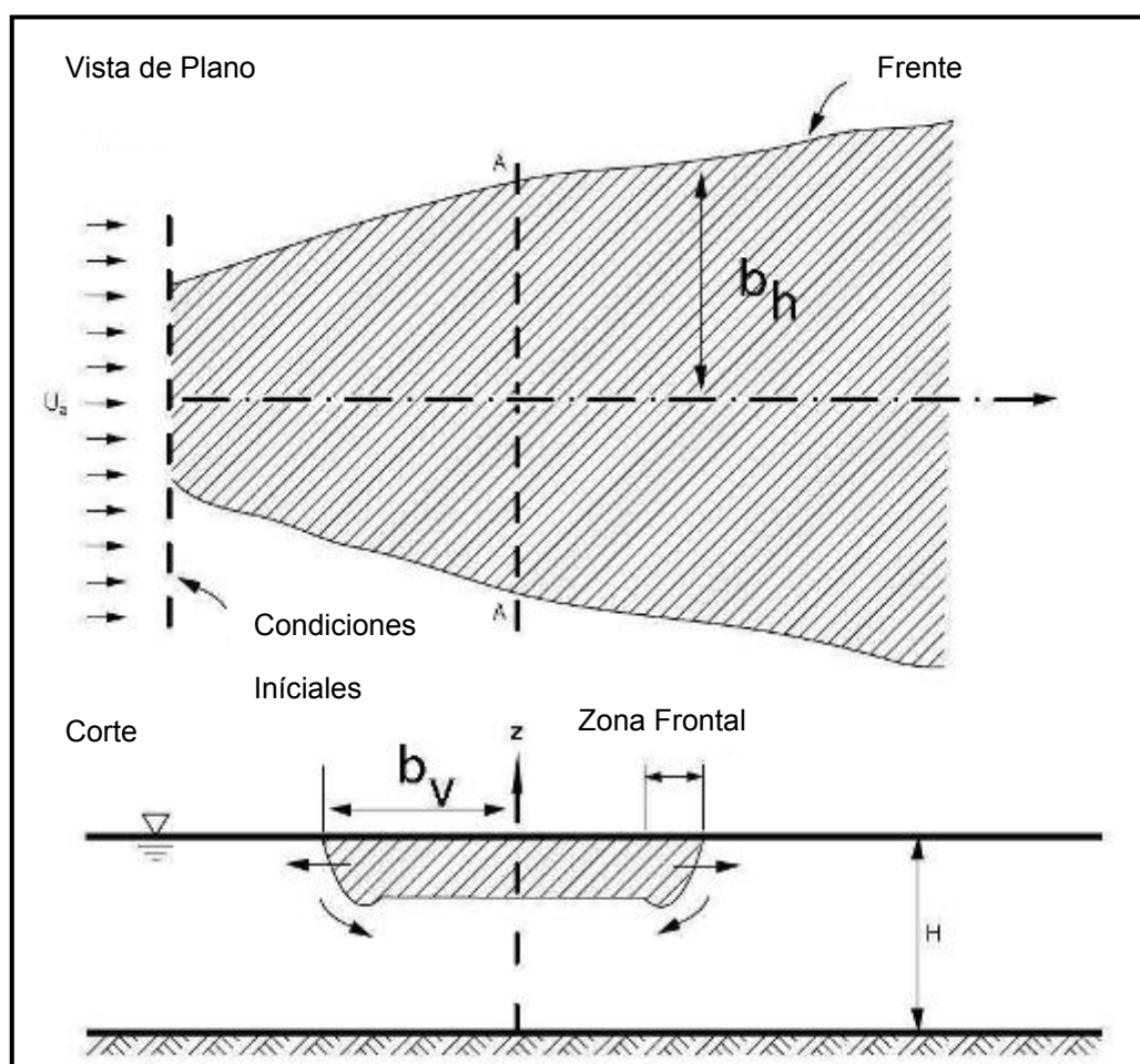
Figura 3.18 Proceso de difusion flotante aguas abajo o cerca de la region de descarga
