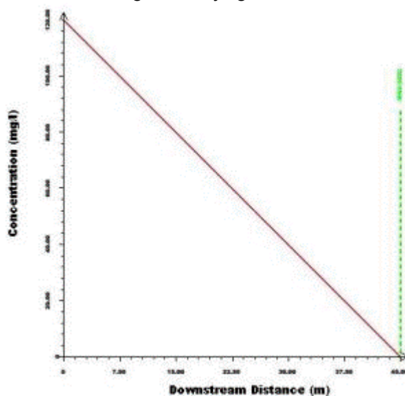
Figura 4.20 CorVue diagrama de concentración vs distancia aguas abajo grilla 1
