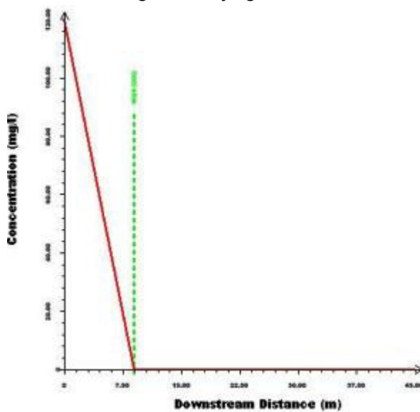
Figura 4.21 CorVue diagrama de concentración vs distancia aguas abajo grilla 5
