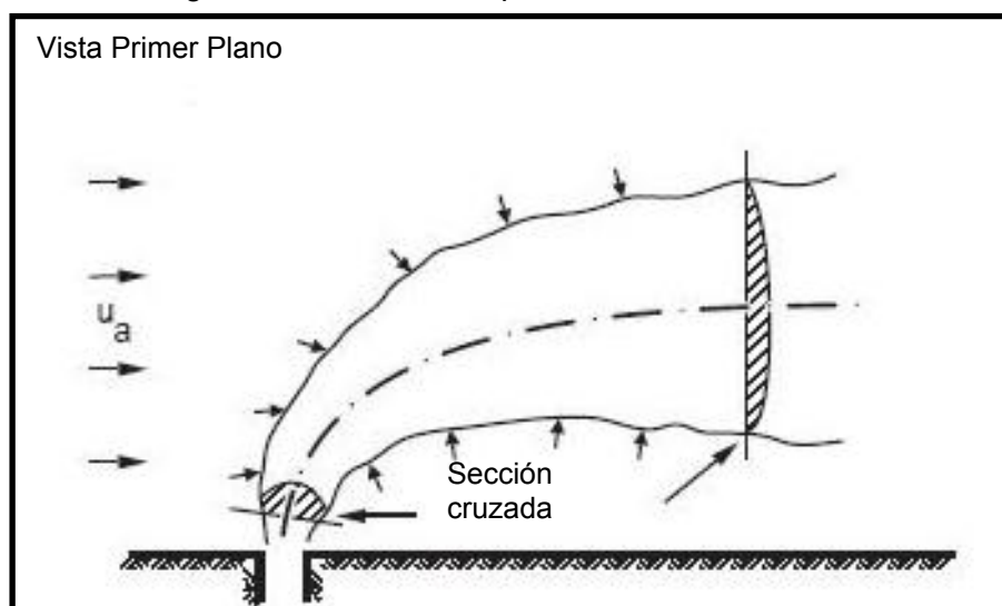
Figura 3.15 Desviación por cruce de corrientes
