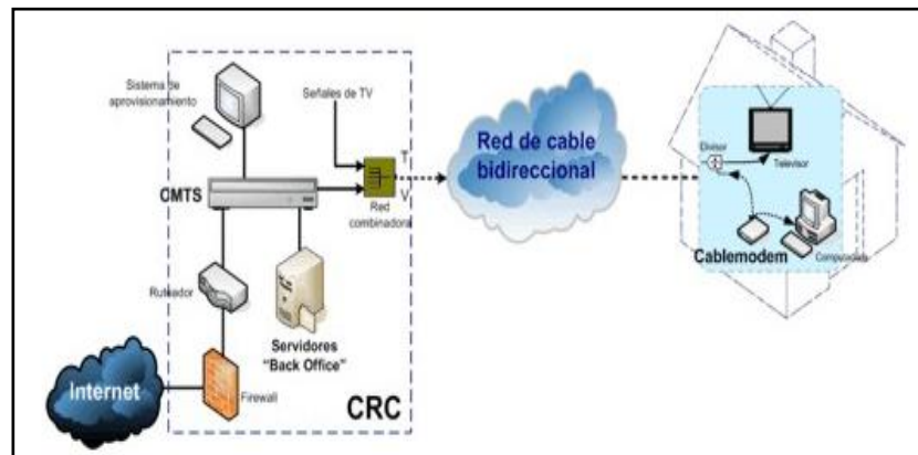
Figura 2.4 Arquitectura de DOCSIS 7
