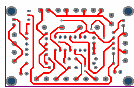
Fig. 4.1.10: Pista superior de la tarjeta Sensor Luz V4.0
