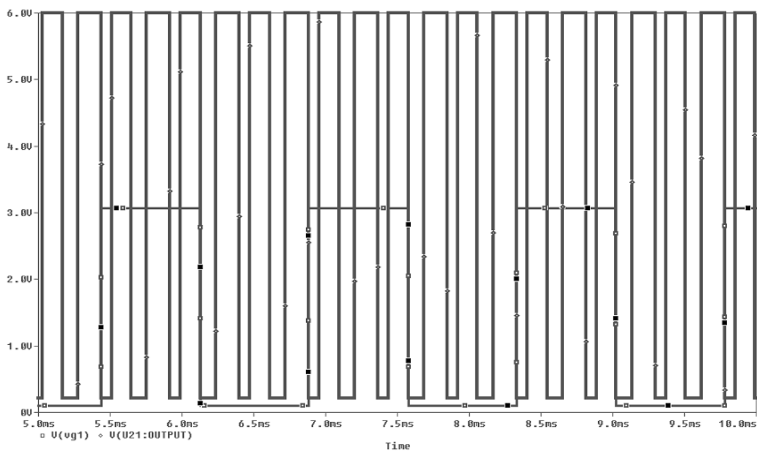
Fig. 5.2 Señal de reloj y desfazamiento (simulación)
