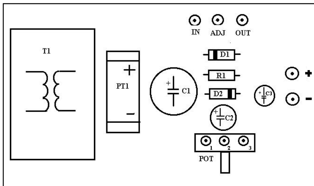
Fig. A.14 Diseño de la Fuente a usar
