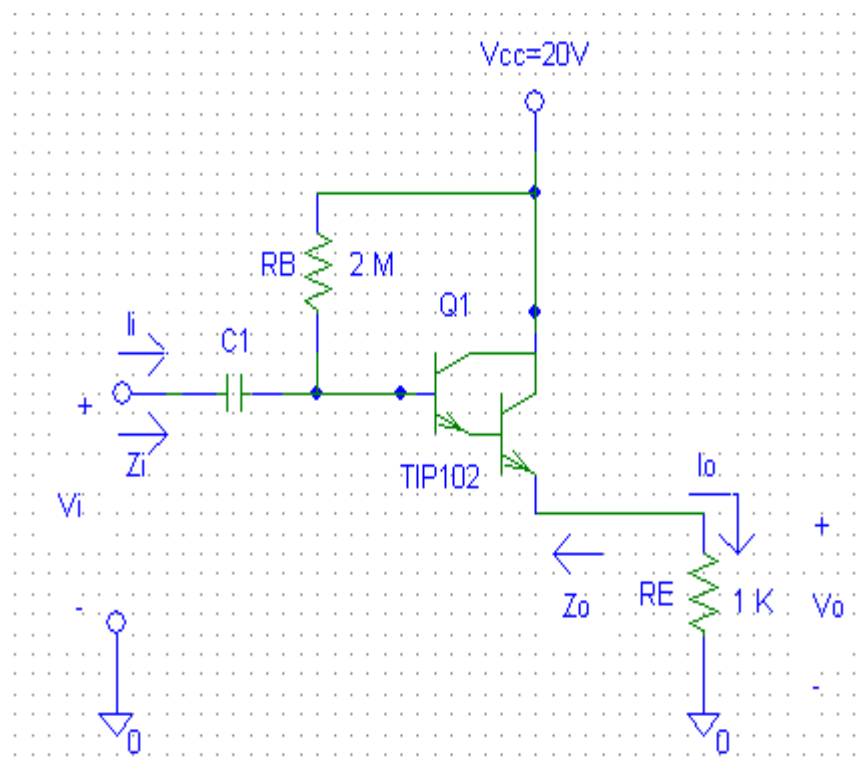
Fig. 2.7 Configuración Darlington
