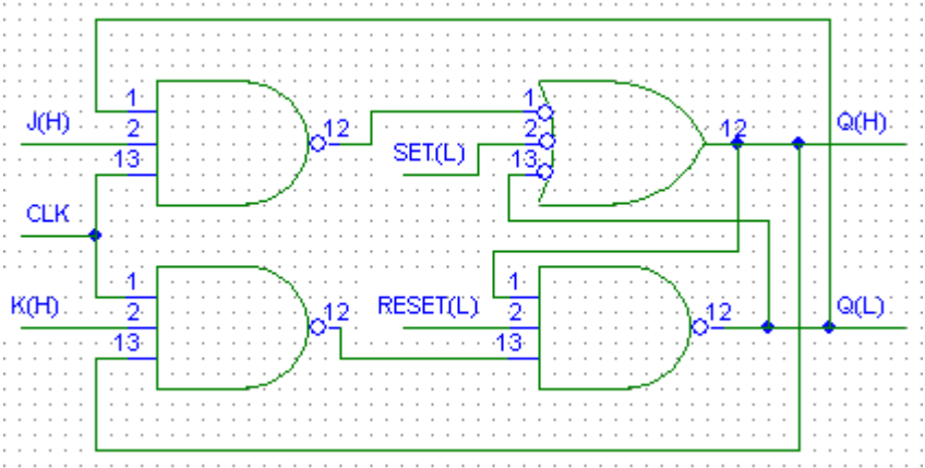
Fig. 3.17 Diagrama Lógico
