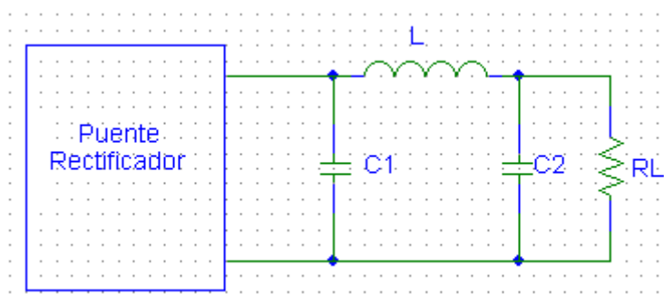
Fig. A.10 Topología del filtro pi L-C
