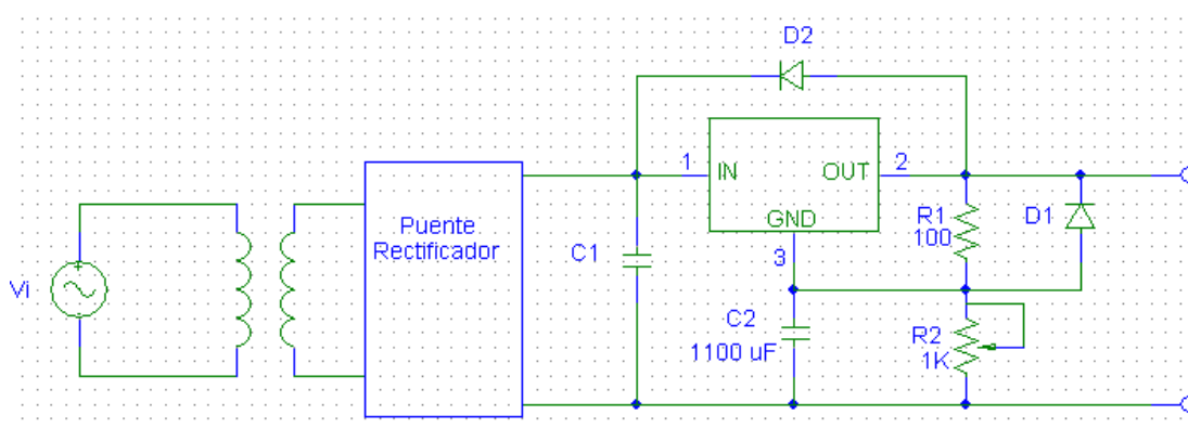
Fig. A.12 Fuente de voltaje Regulada
