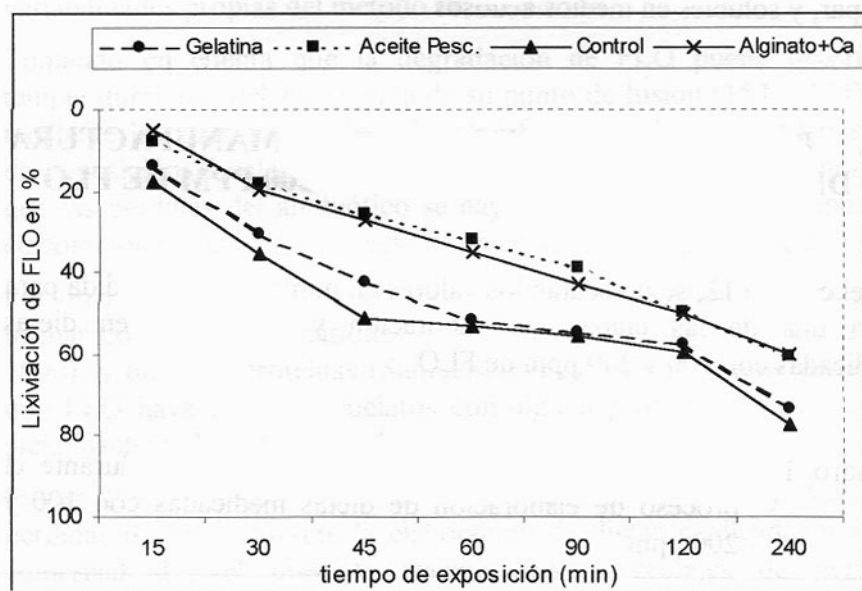
Figura 6. Pérdidas en % de lixiviación de tres recubridores durante cuatro horas de exposición en agua de mar
