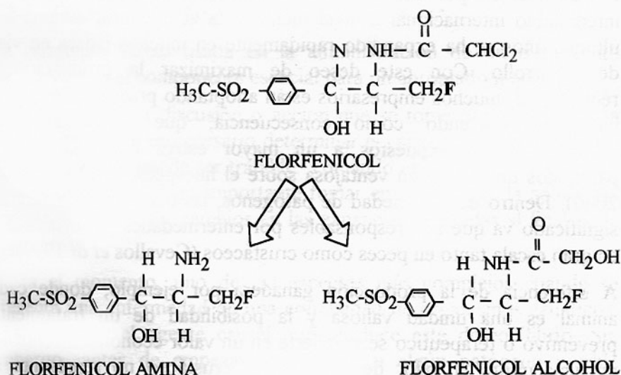
Figura 3. Estructura química de florfenicol y sus metabolitos florfenicol amina y florfenicol alcohol.
