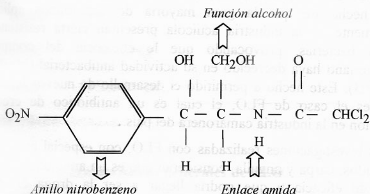
Figura 1. Estructura química del Cloranfenicol
