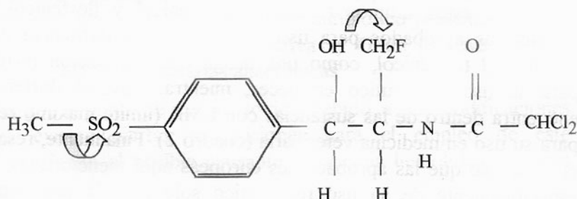
Figura 2. Estructura química del Florfenicol y sus modificaciones
