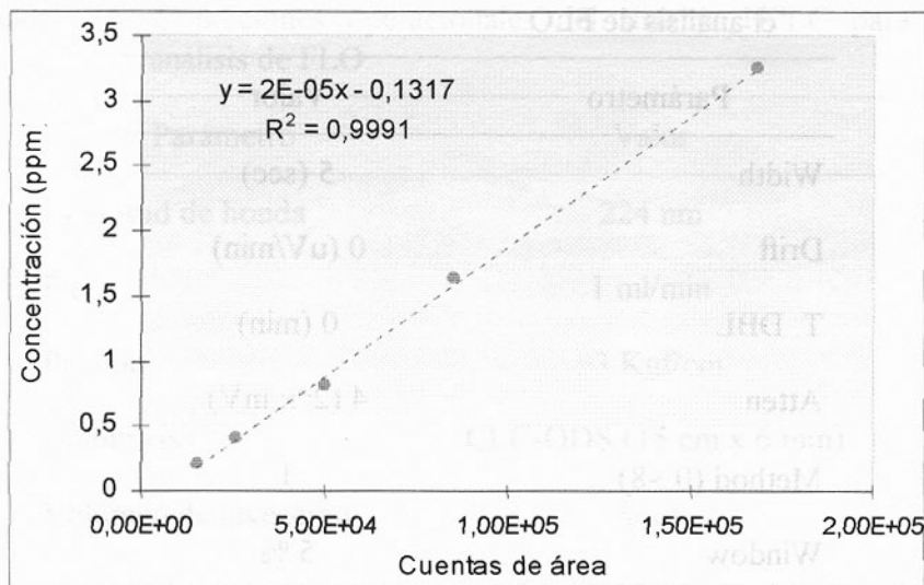
Figura 11. Curva de calibración para FLO de acuerdo a las condiciones analíticas establecidas
