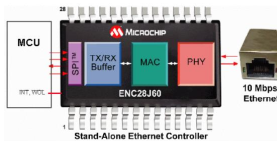
Figura 6. Módulo ENC28J60
